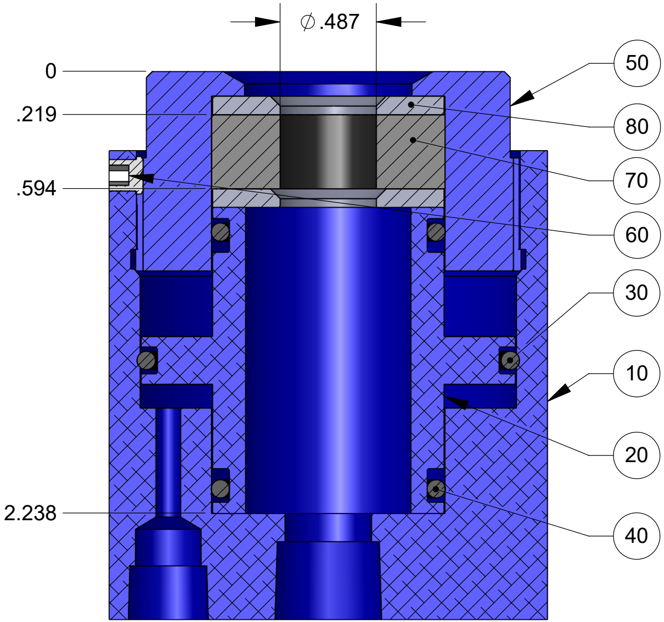
SECTION A-A
