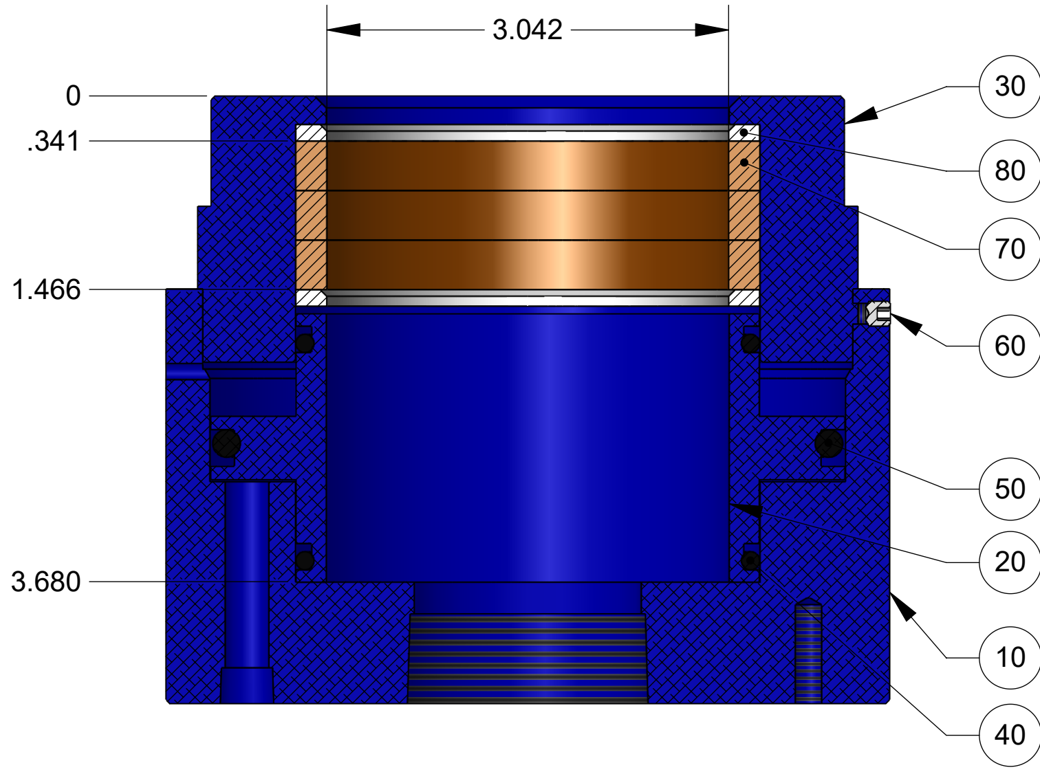
SECTION A-A
