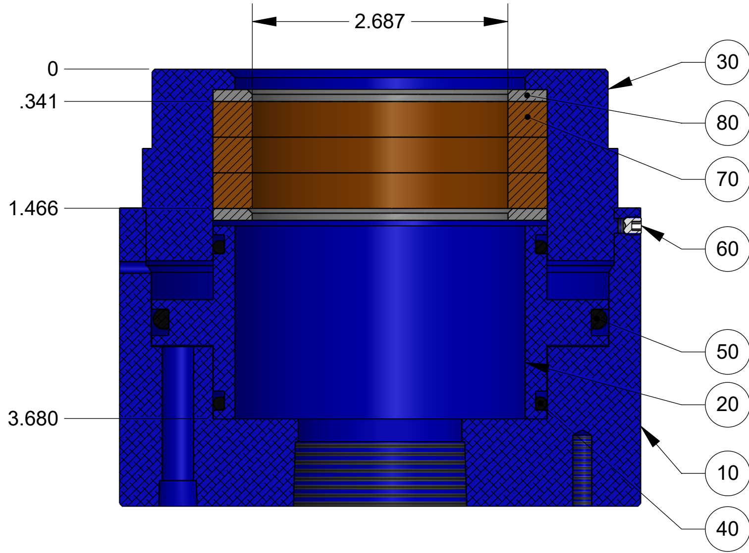
SECTION A-A
