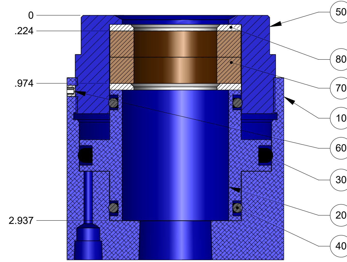
SECTION A-A SCALE 3 : 2
