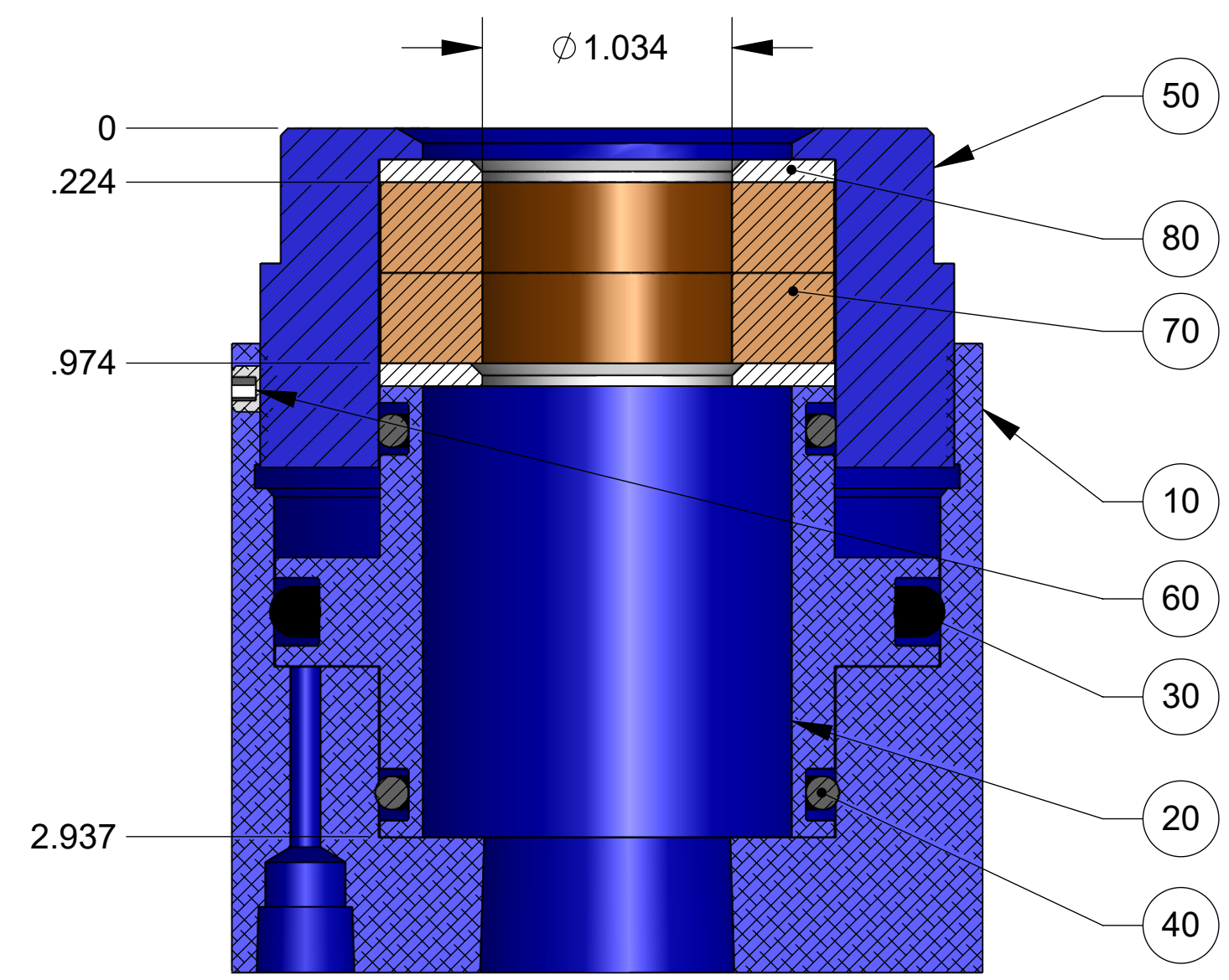
SECTION A-A SCALE 3 : 2
