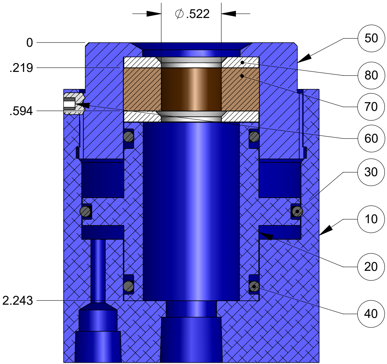
SECTION A-A
