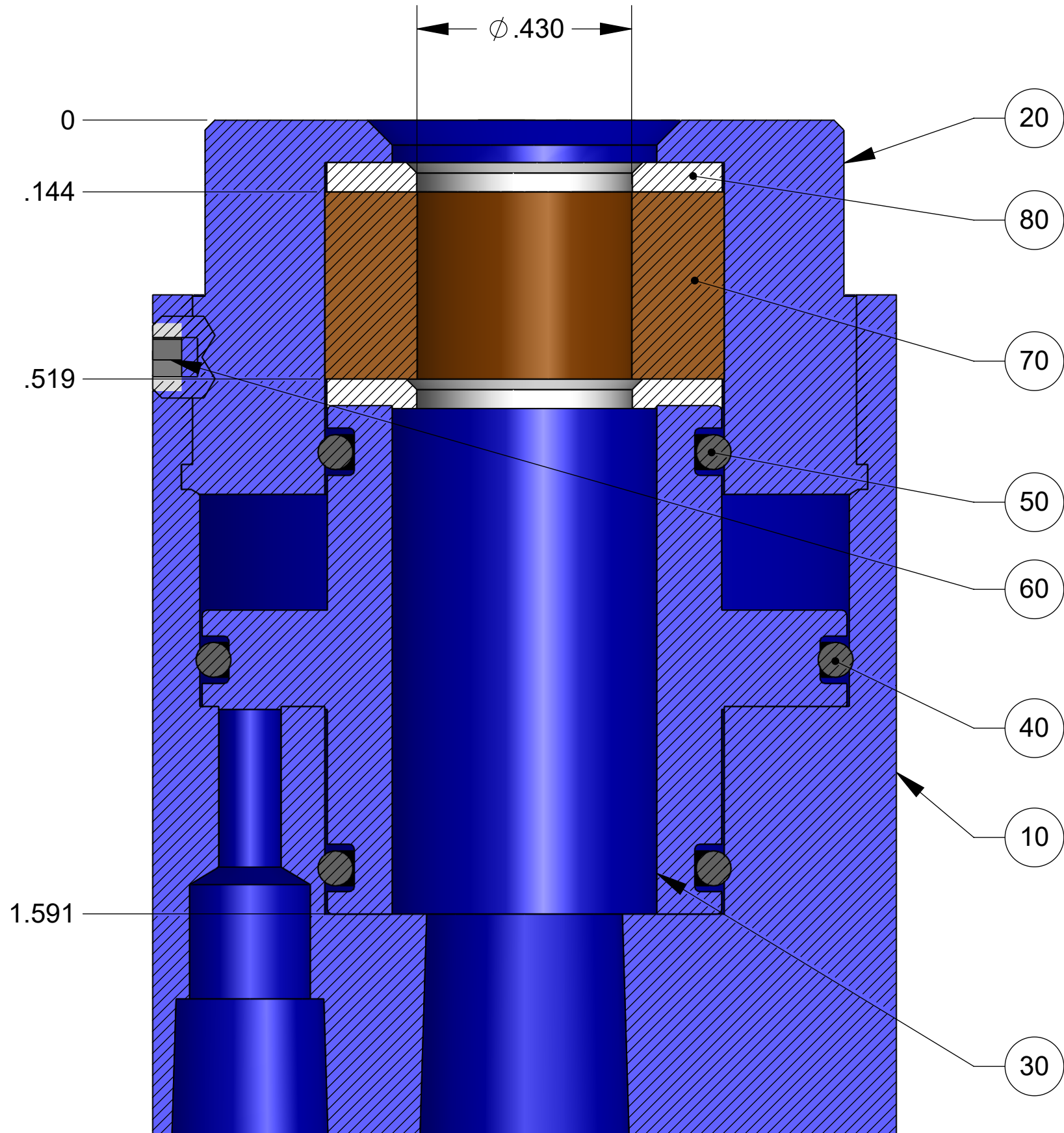
SECTION A-A
