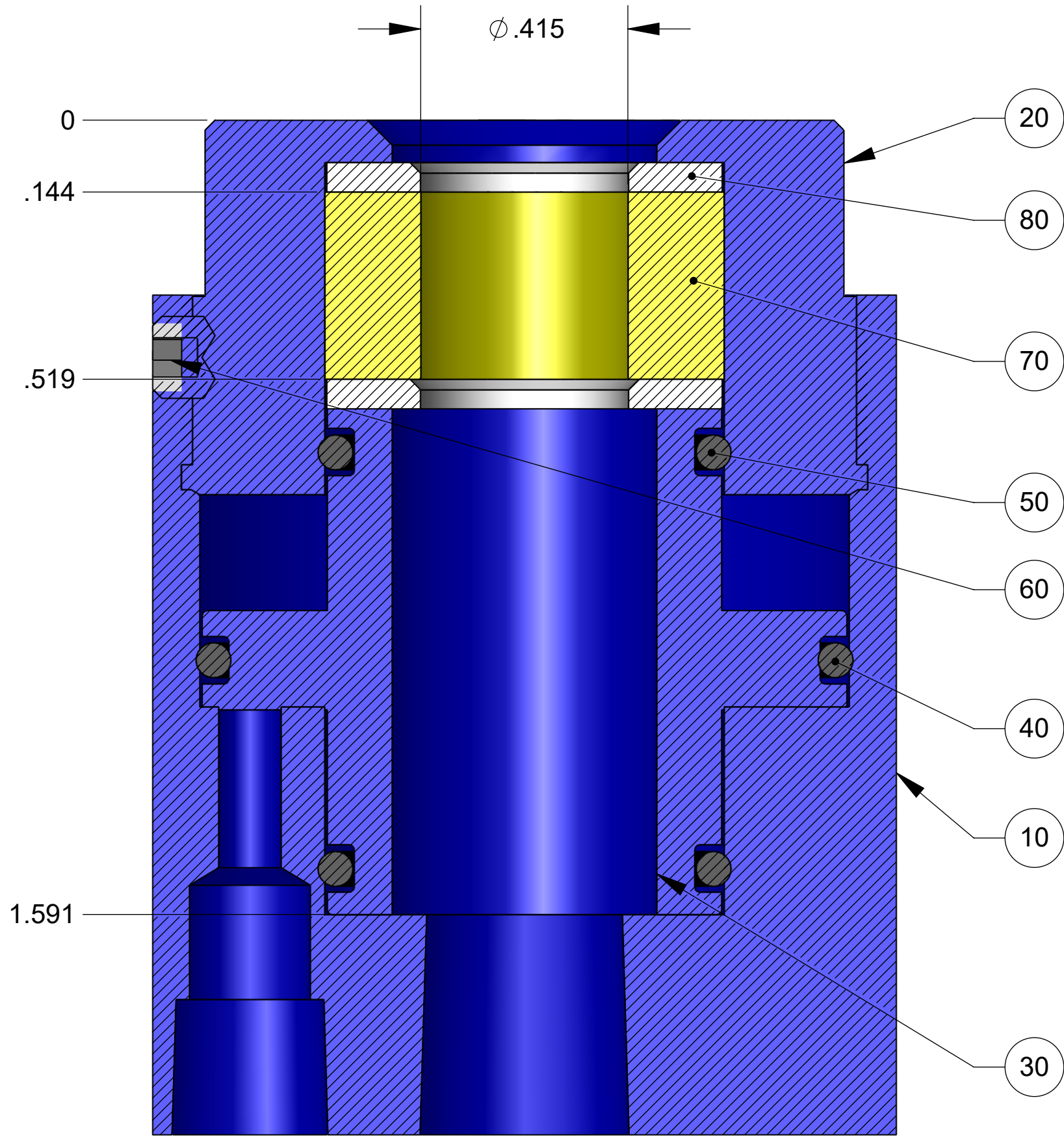
SECTION A-A
