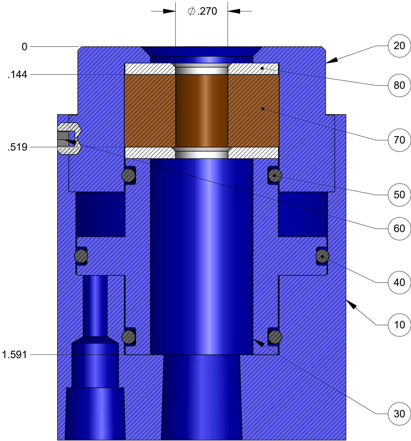
SECTION A-A
