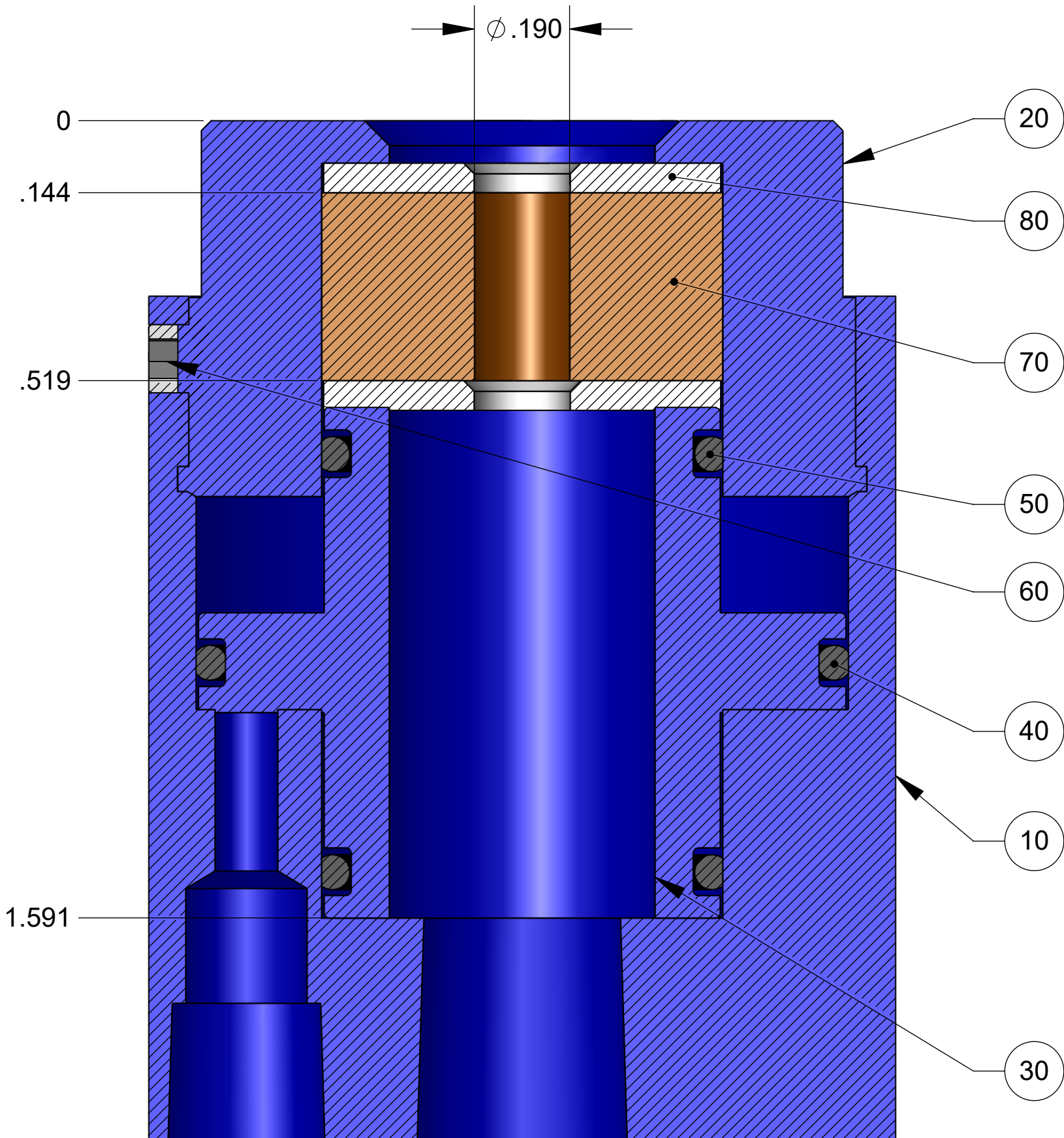
SECTION A-A
