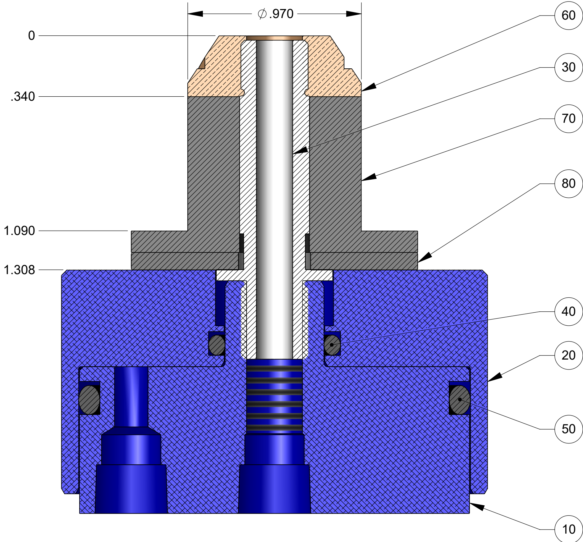
SECTION A-A SCALE 3 : 1
