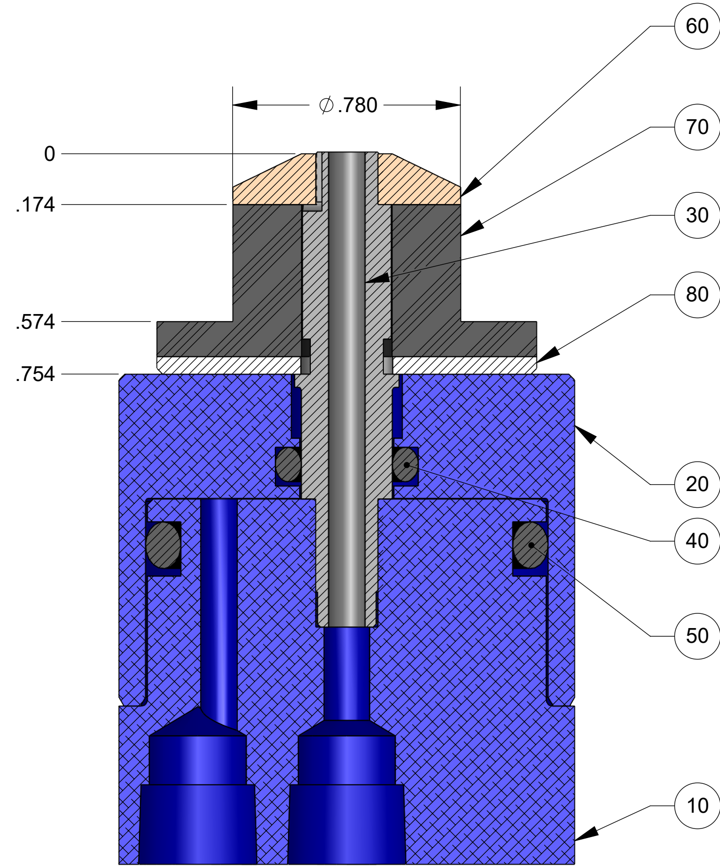
SECTION A-A SCALE 3 : 1
