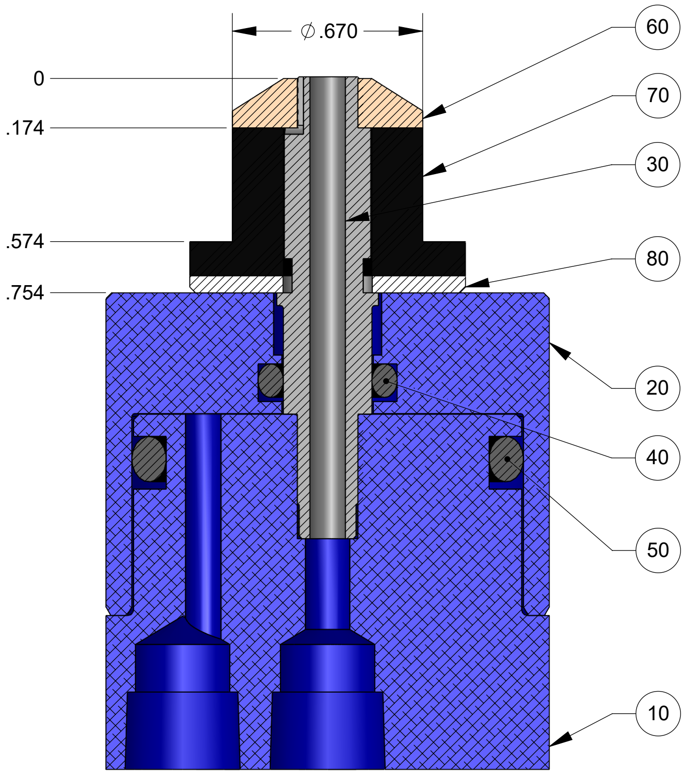
SECTION A-A SCALE 3 : 1
