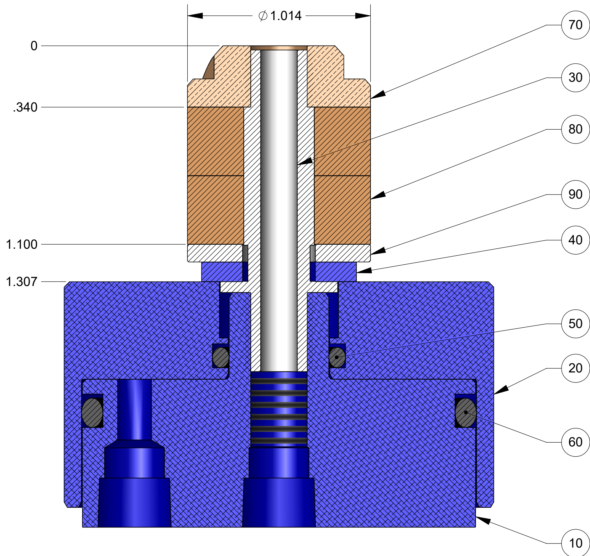
SECTION A-A SCALE 3 : 1
