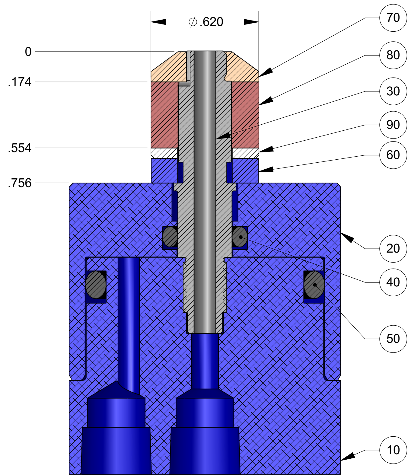
SECTION A-A SCALE 3 : 1
