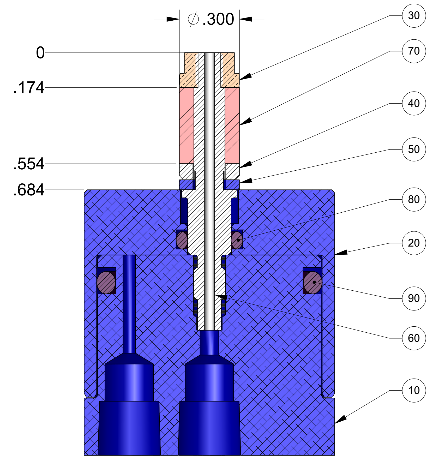
SECTION A-A SCALE 4 : 1
