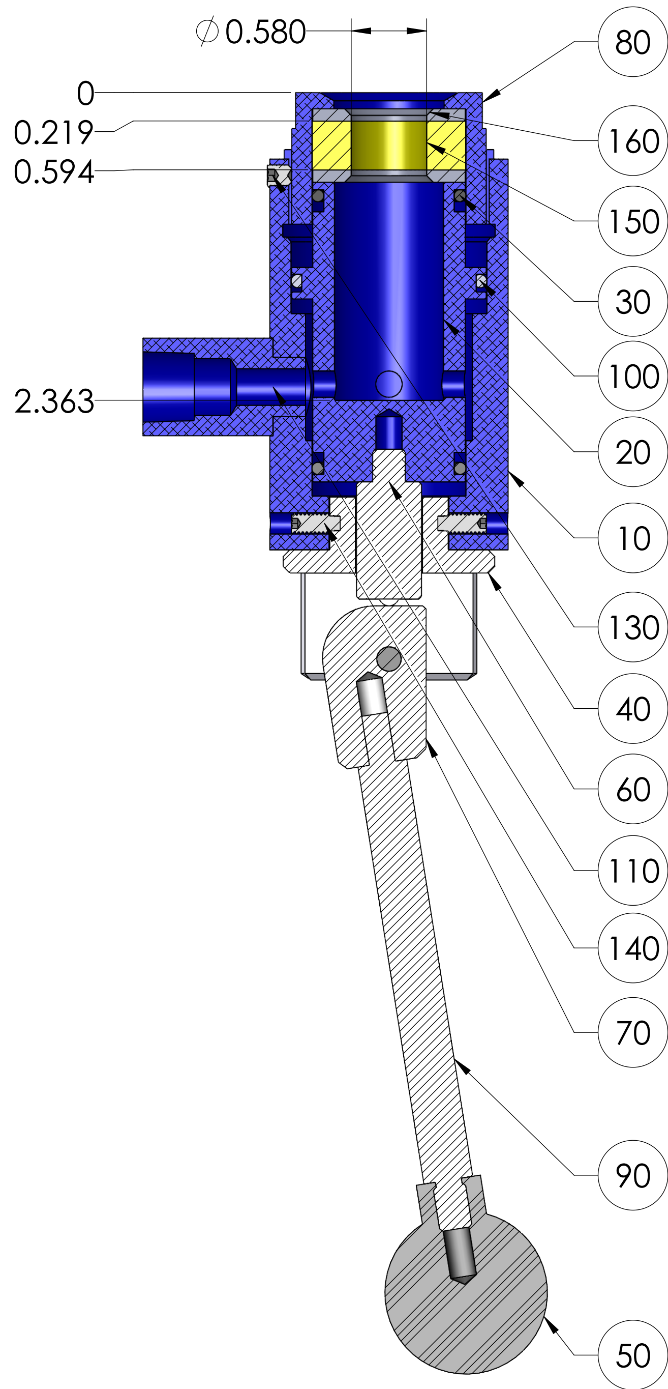
SECTION A-A SCALE 4 : 3
