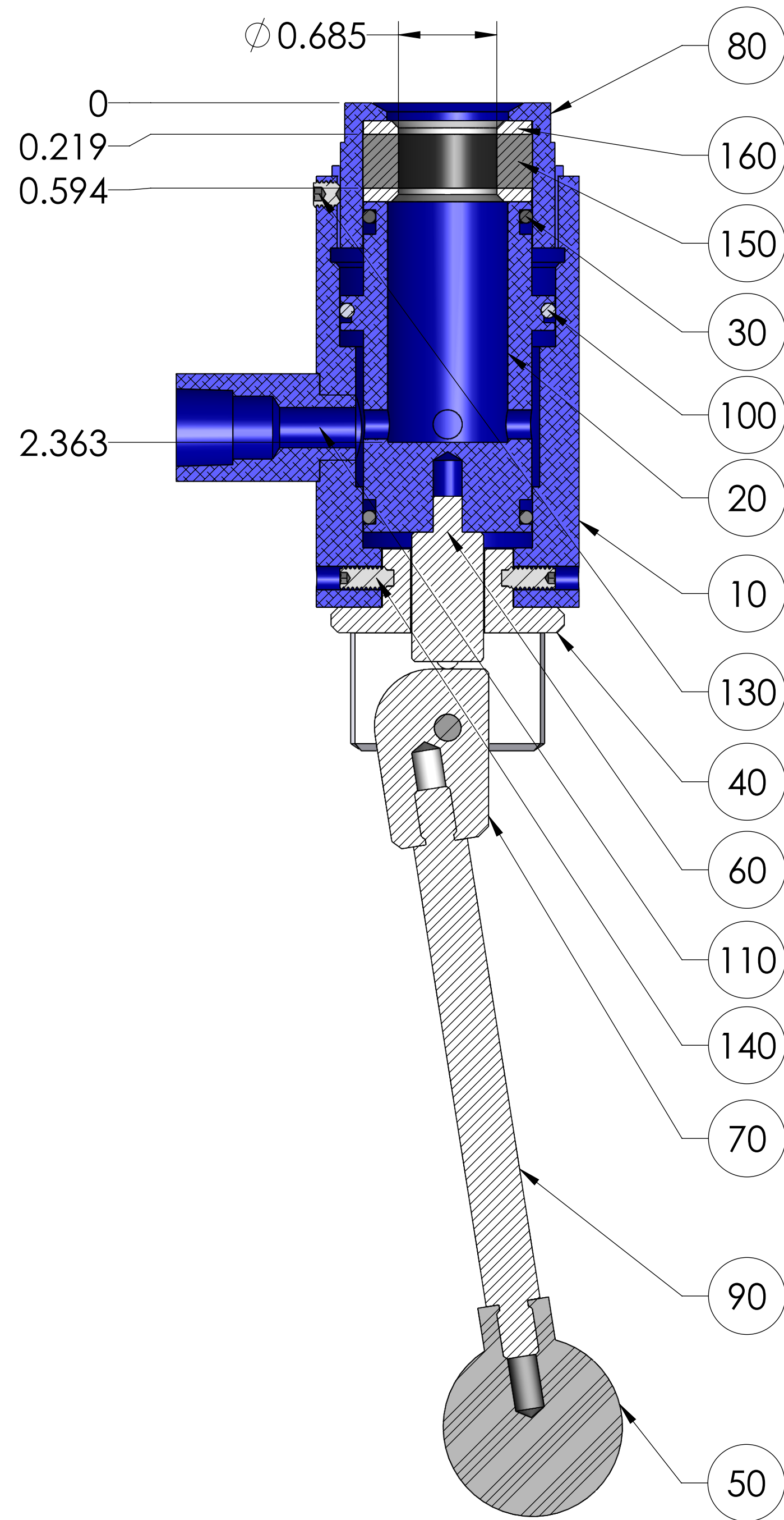
SECTION A-A SCALE 4 : 3
