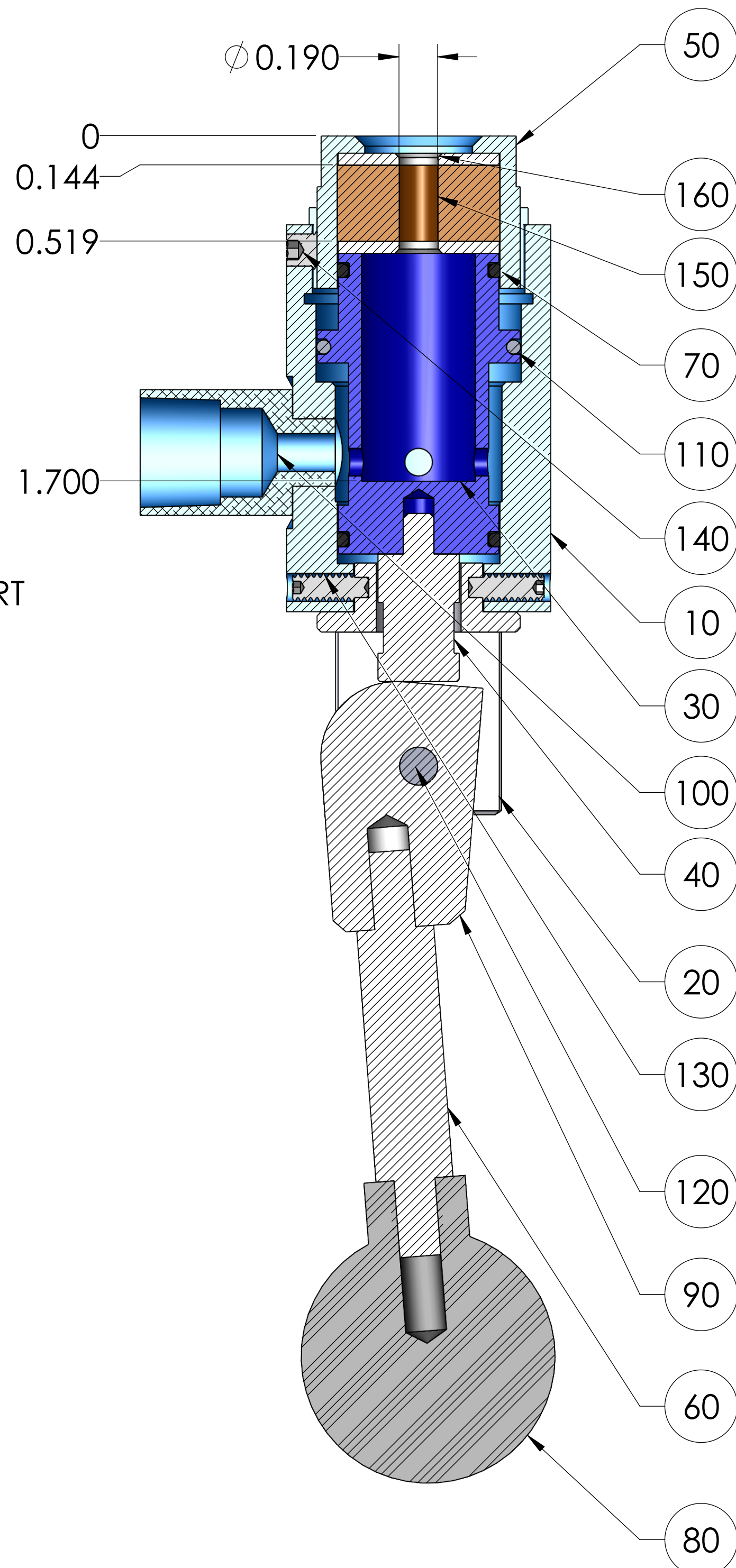
SECTION A-A SCALE 2 : 1
