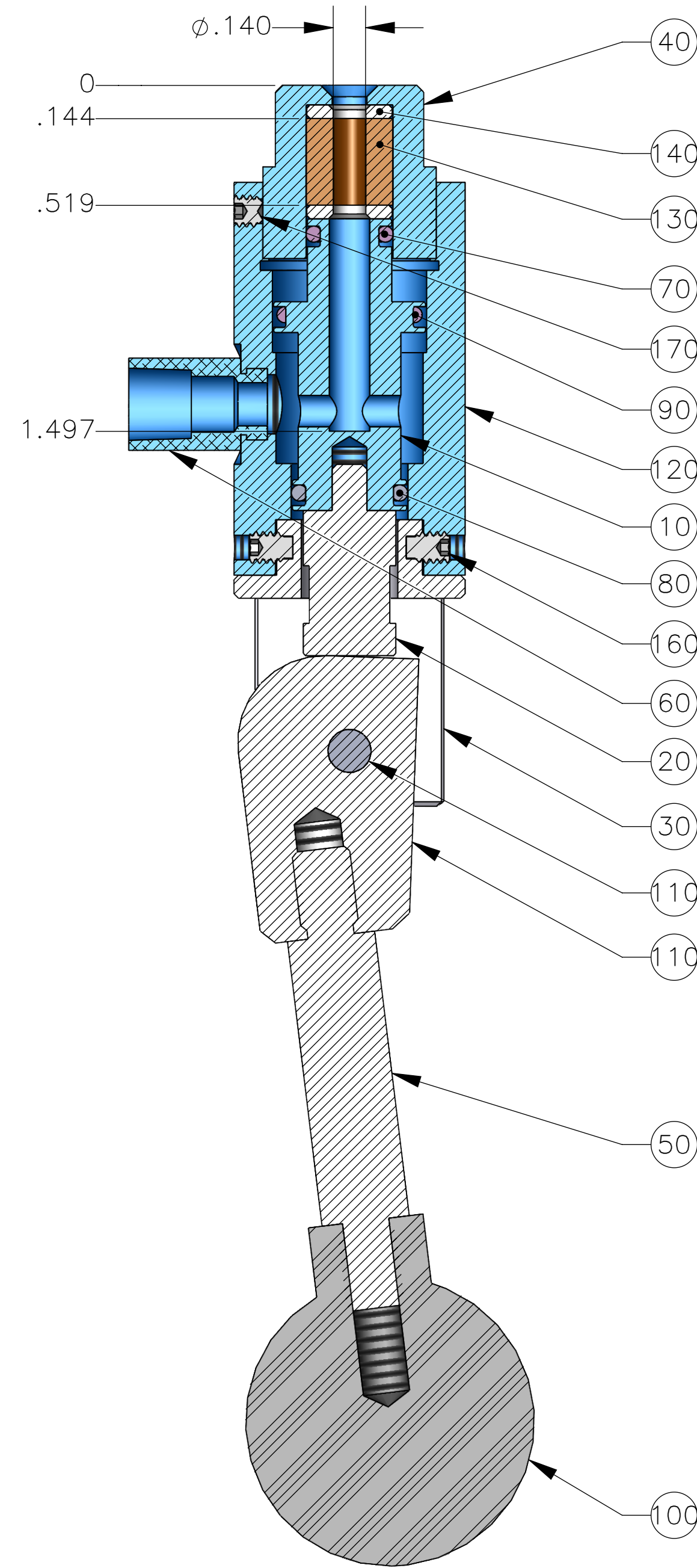
SECTION A-A
