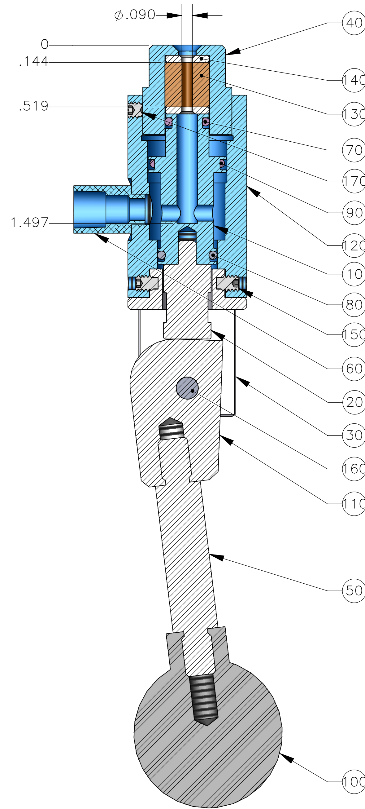
SECTION A-A
