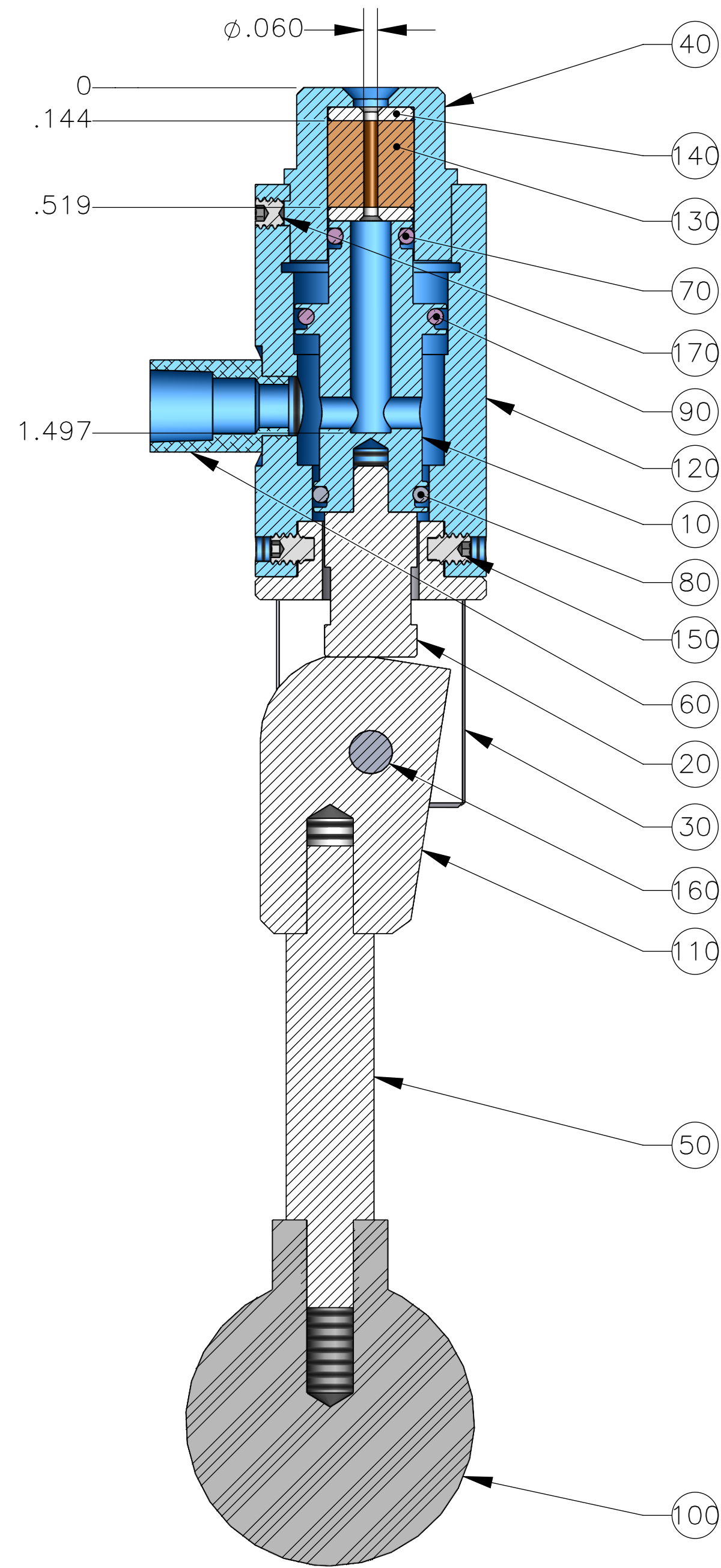
SECTION A-A
