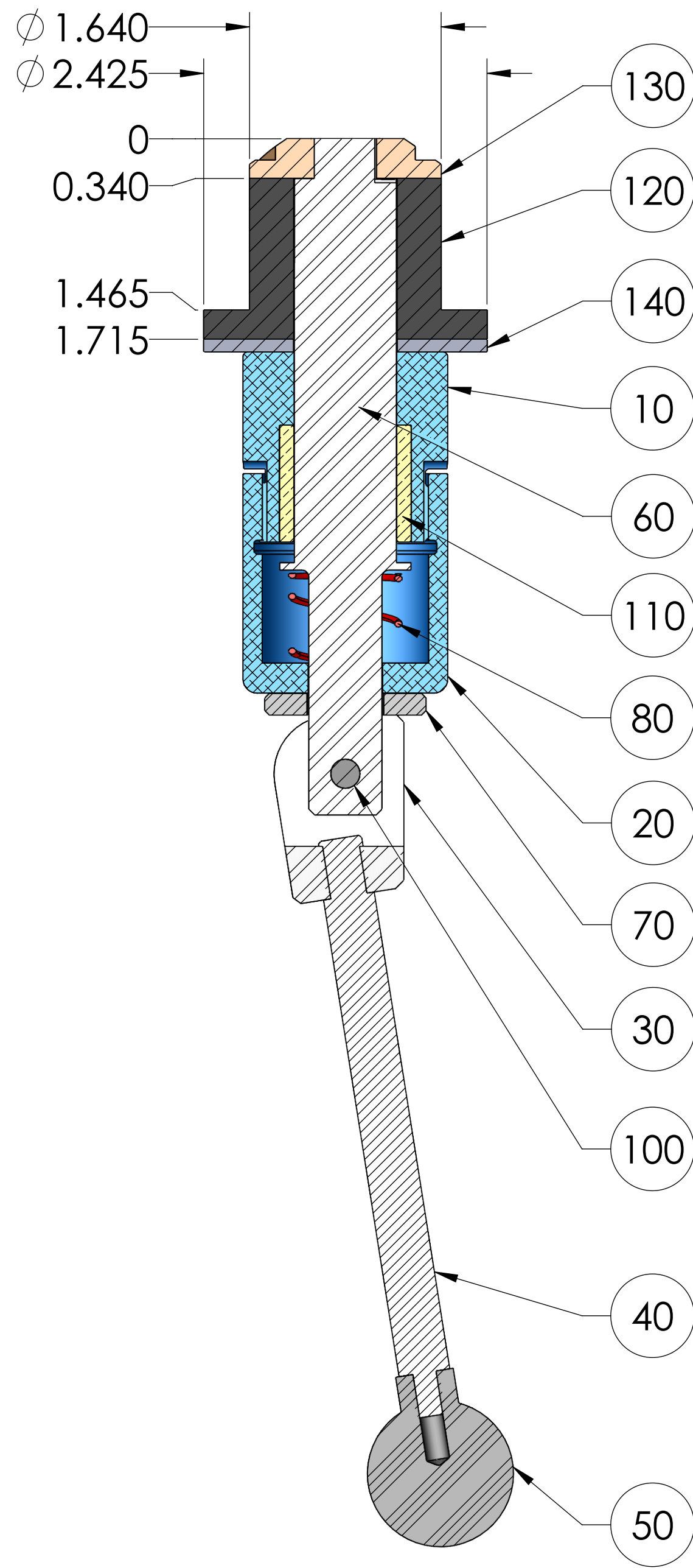
SECTION A-A
