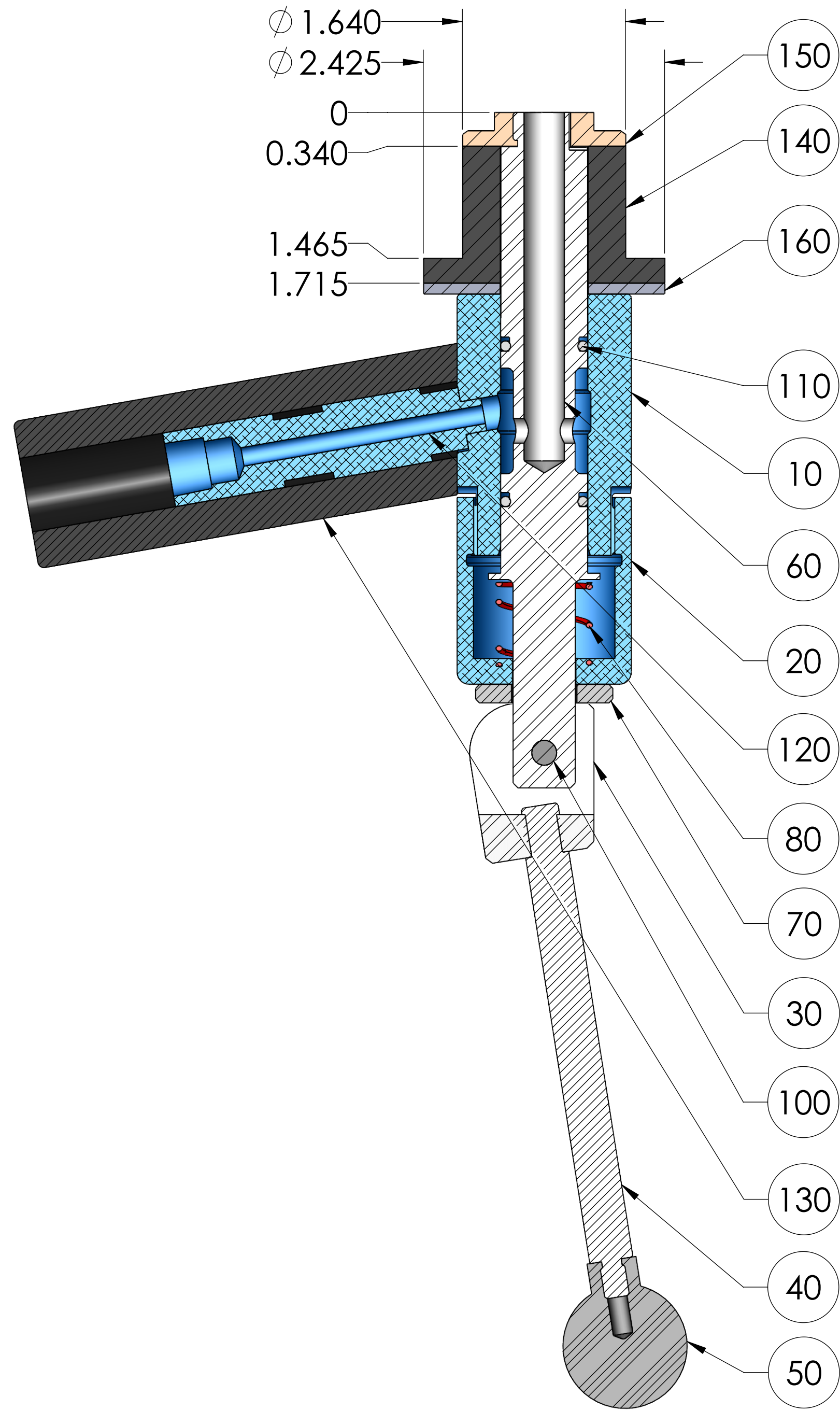
SECTION A-A
