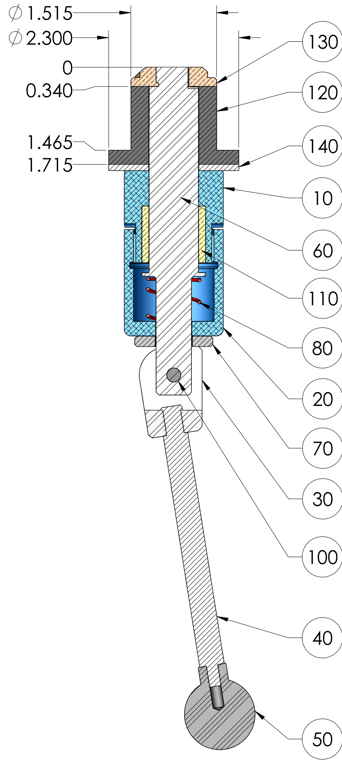
SECTION A-A
