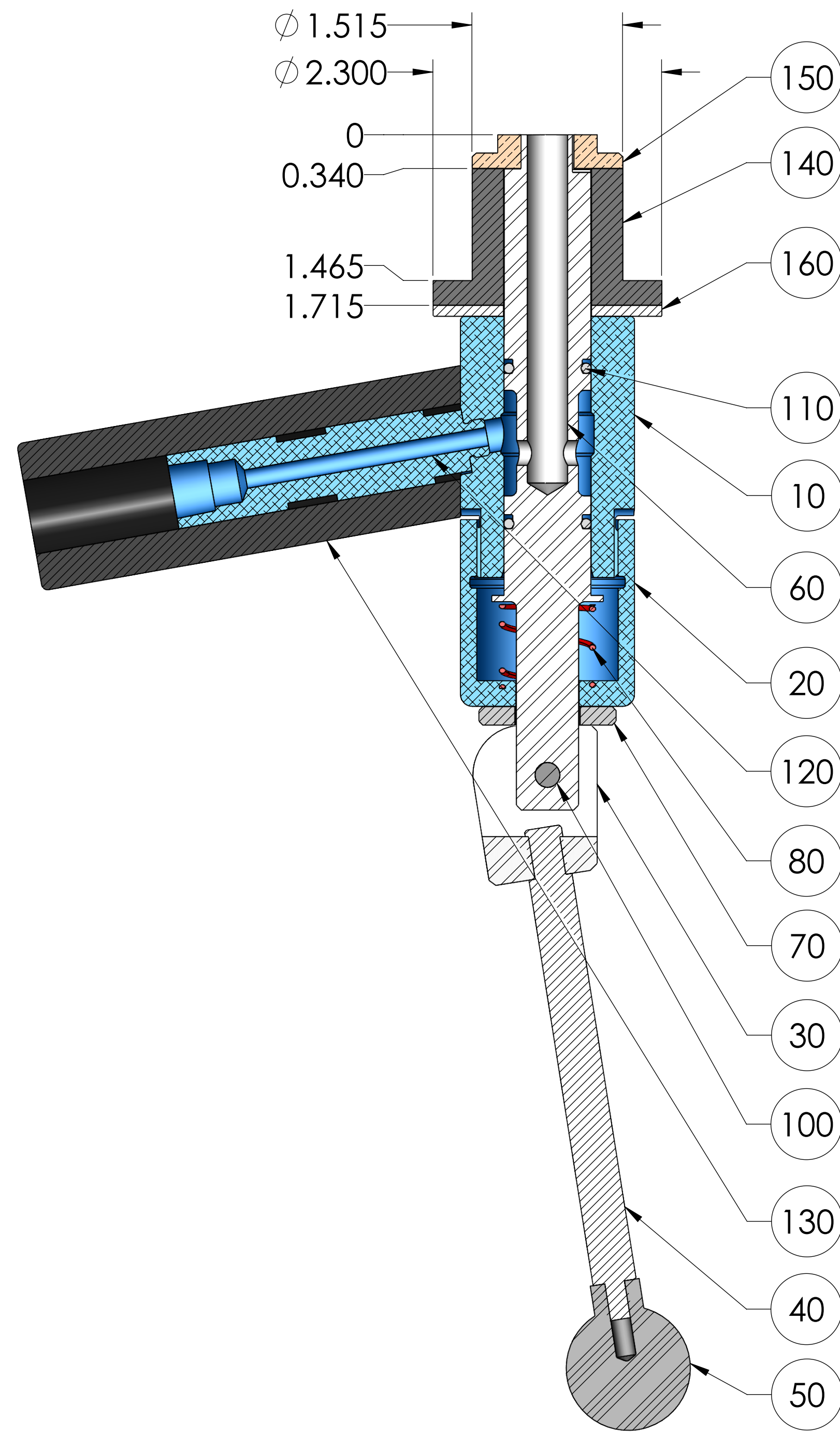
SECTION A-A
