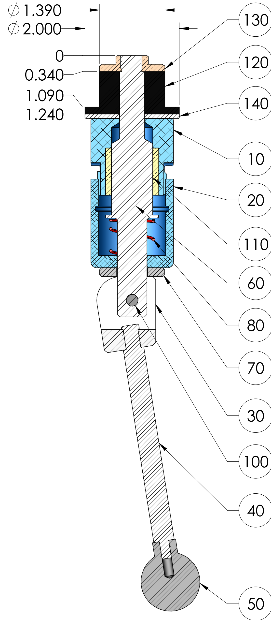
SECTION A-A
