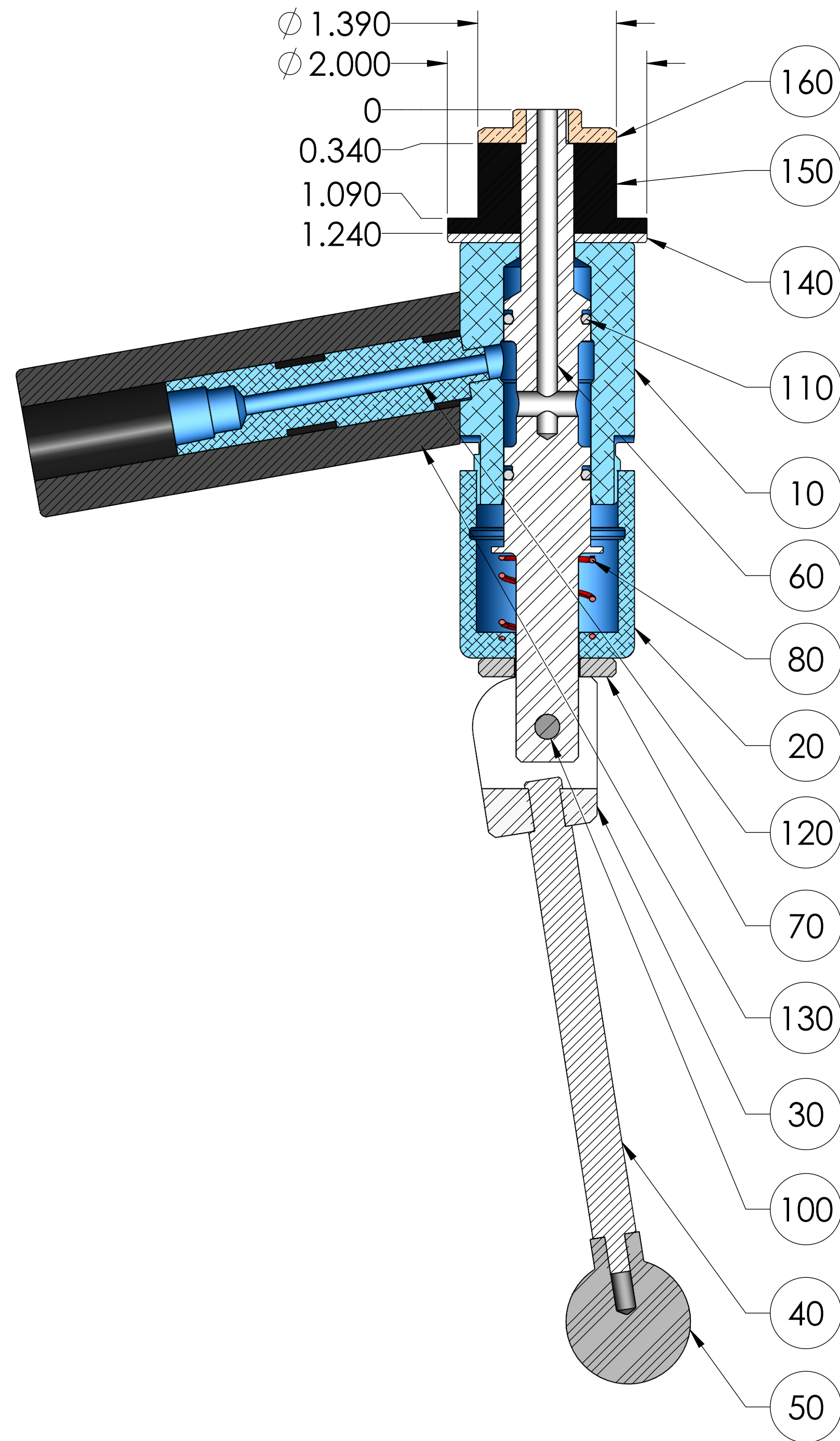
SECTION A-A
