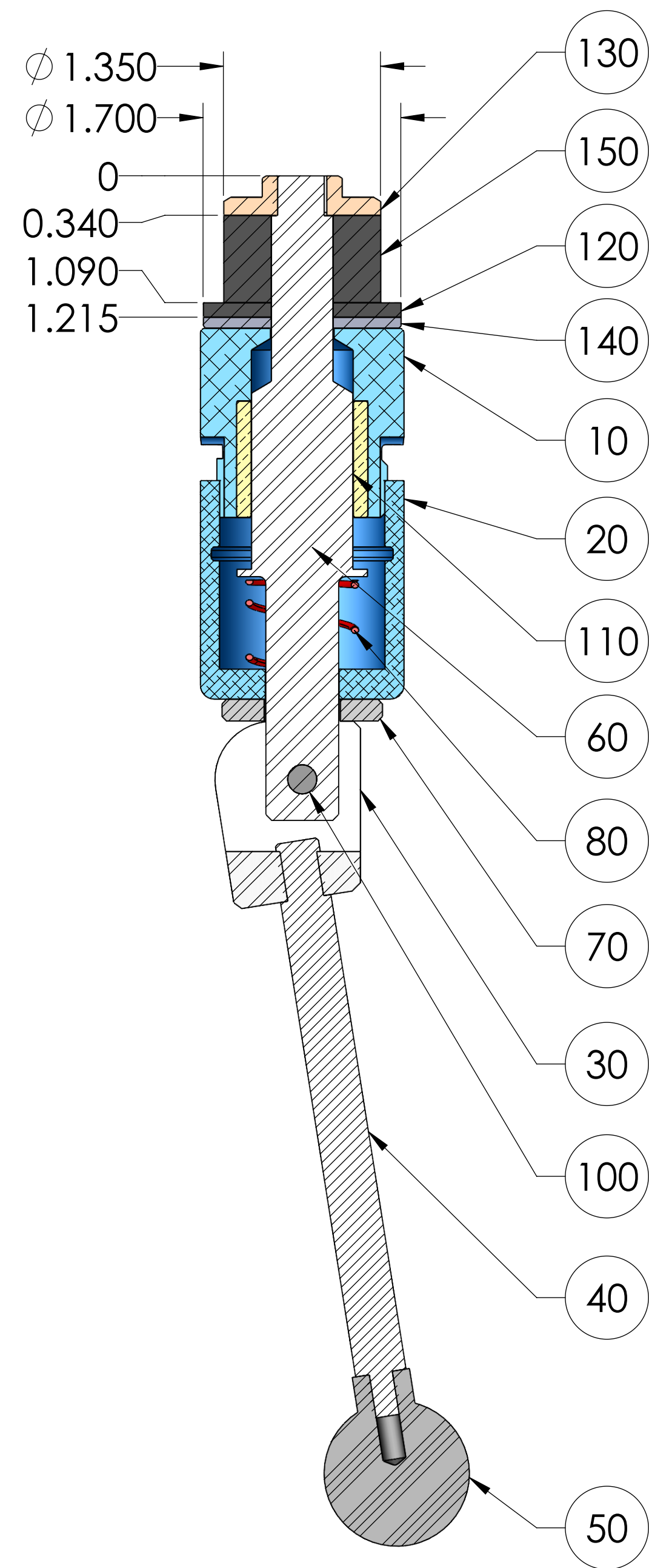
SECTION A-A
