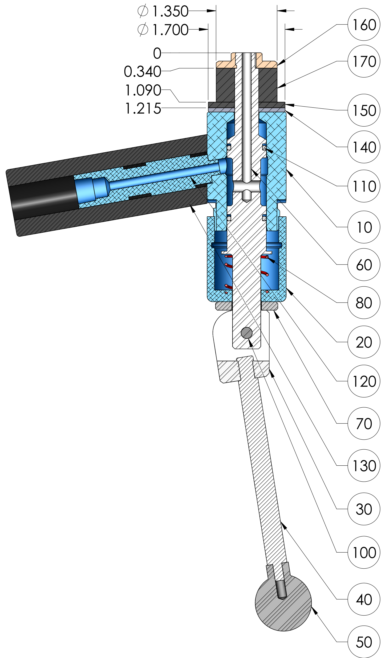
SECTION A-A
