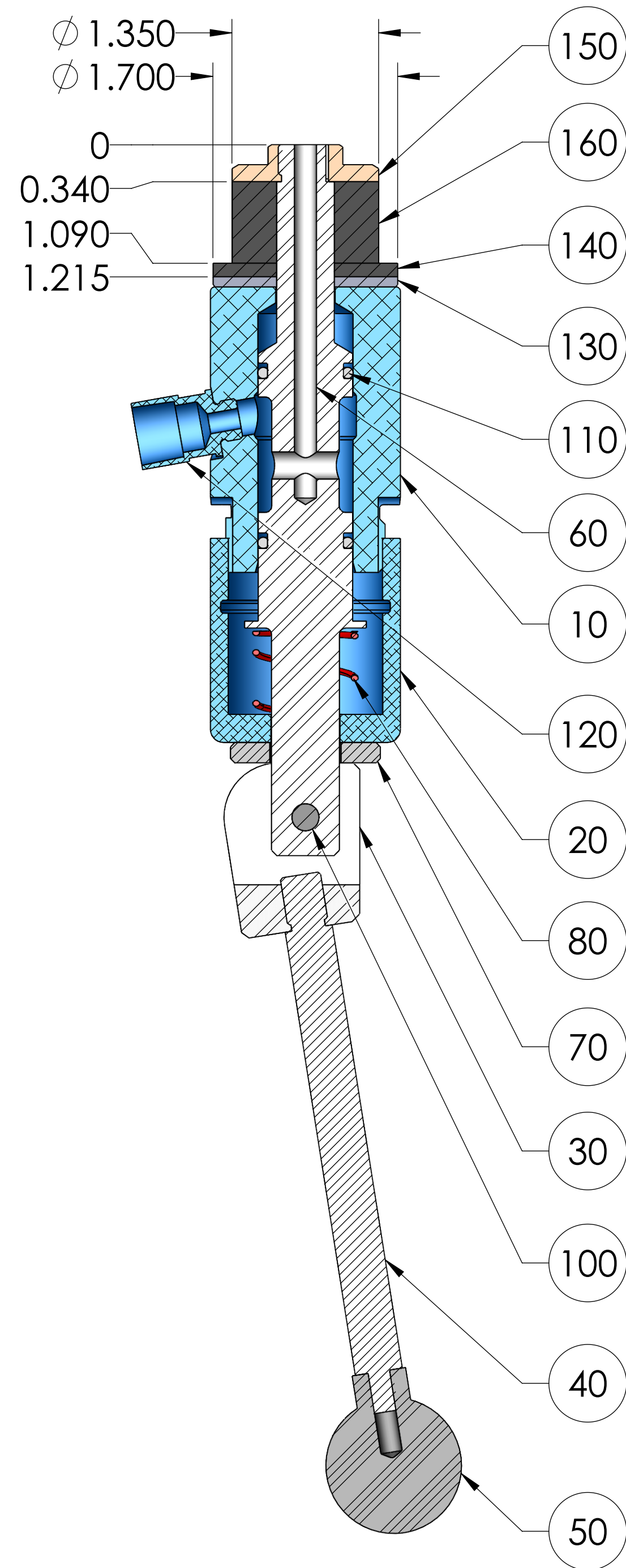
SECTION A-A
