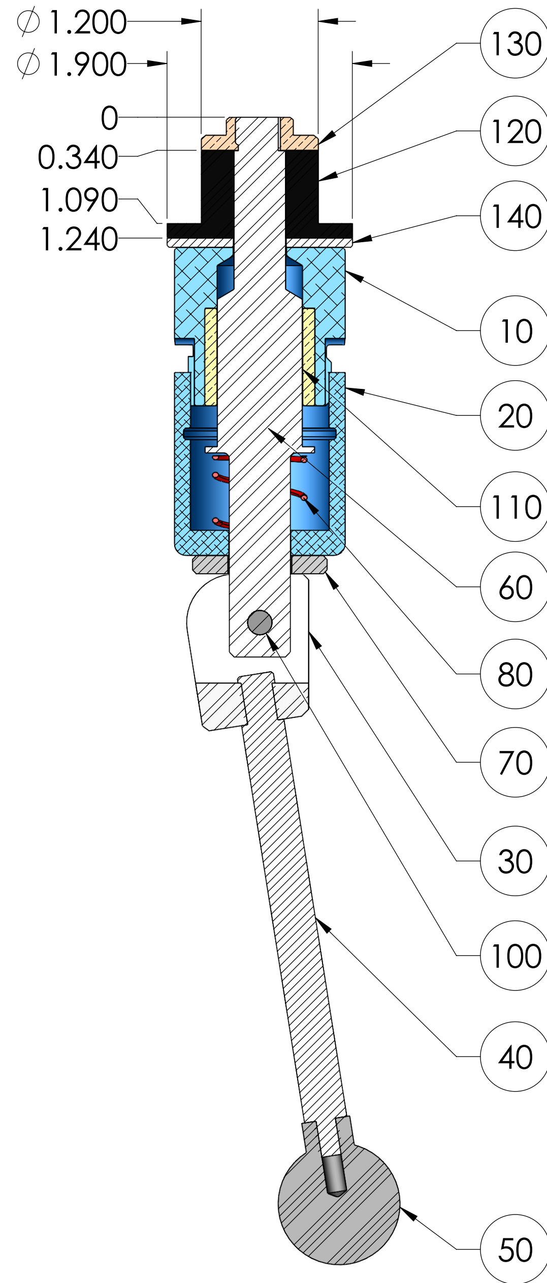
SECTION A-A
