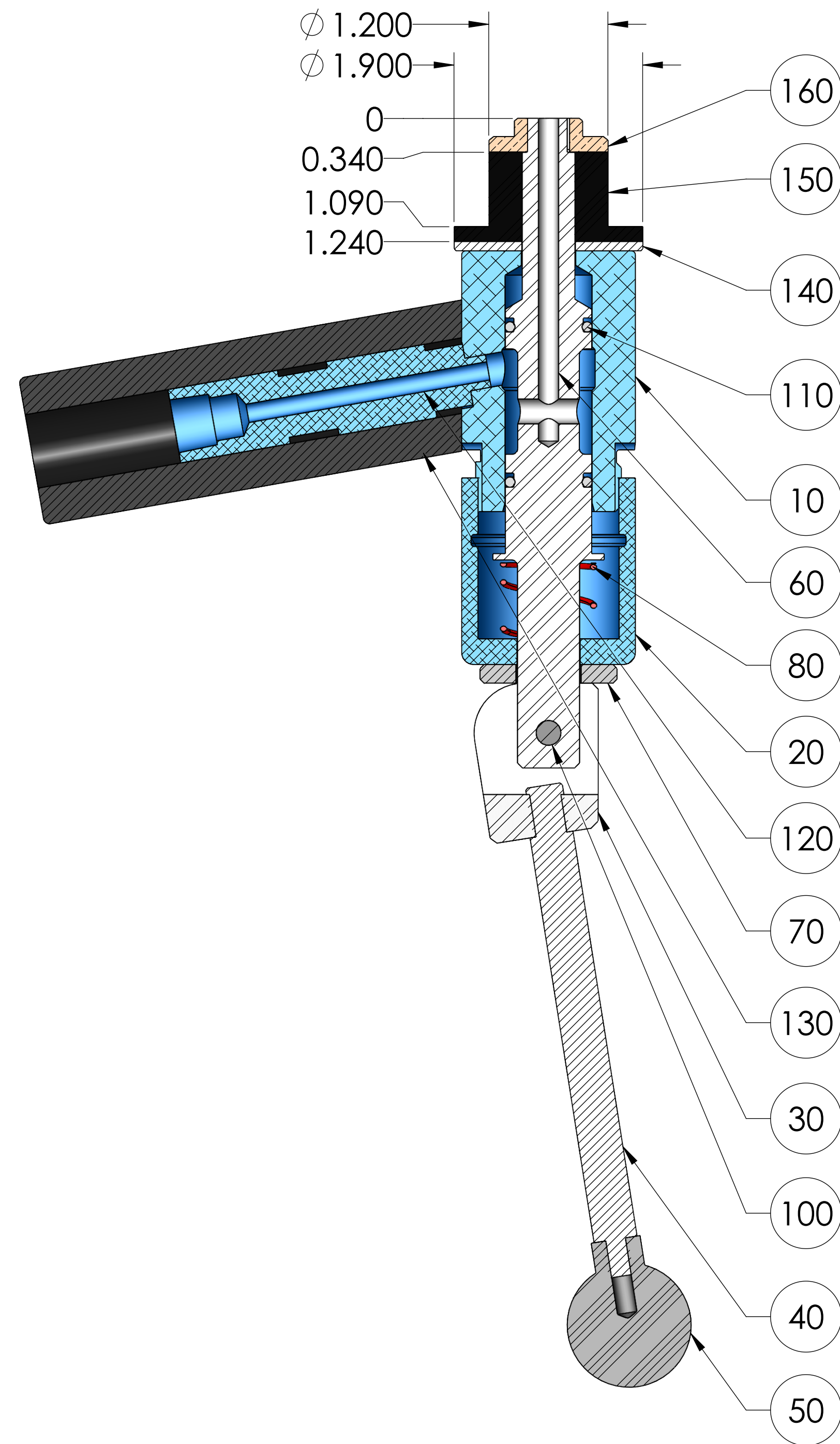
SECTION A-A
