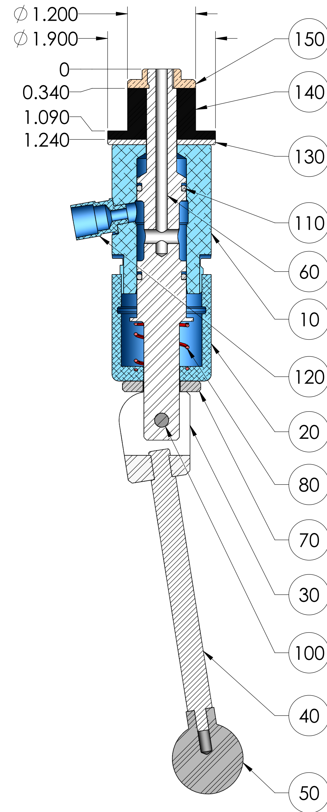
SECTION A-A
