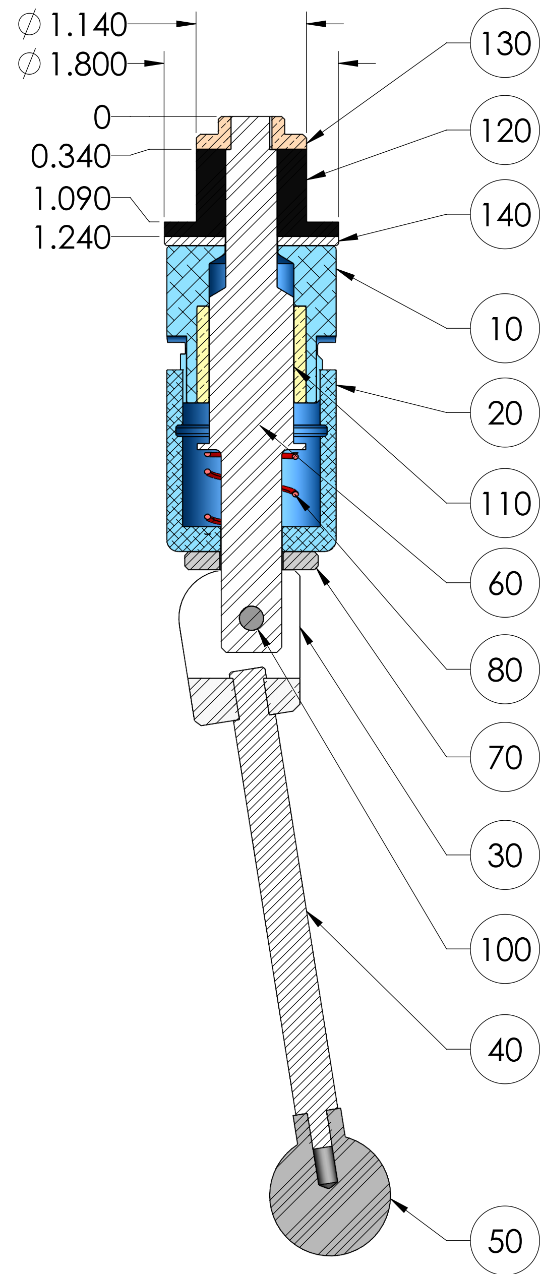
SECTION A-A
