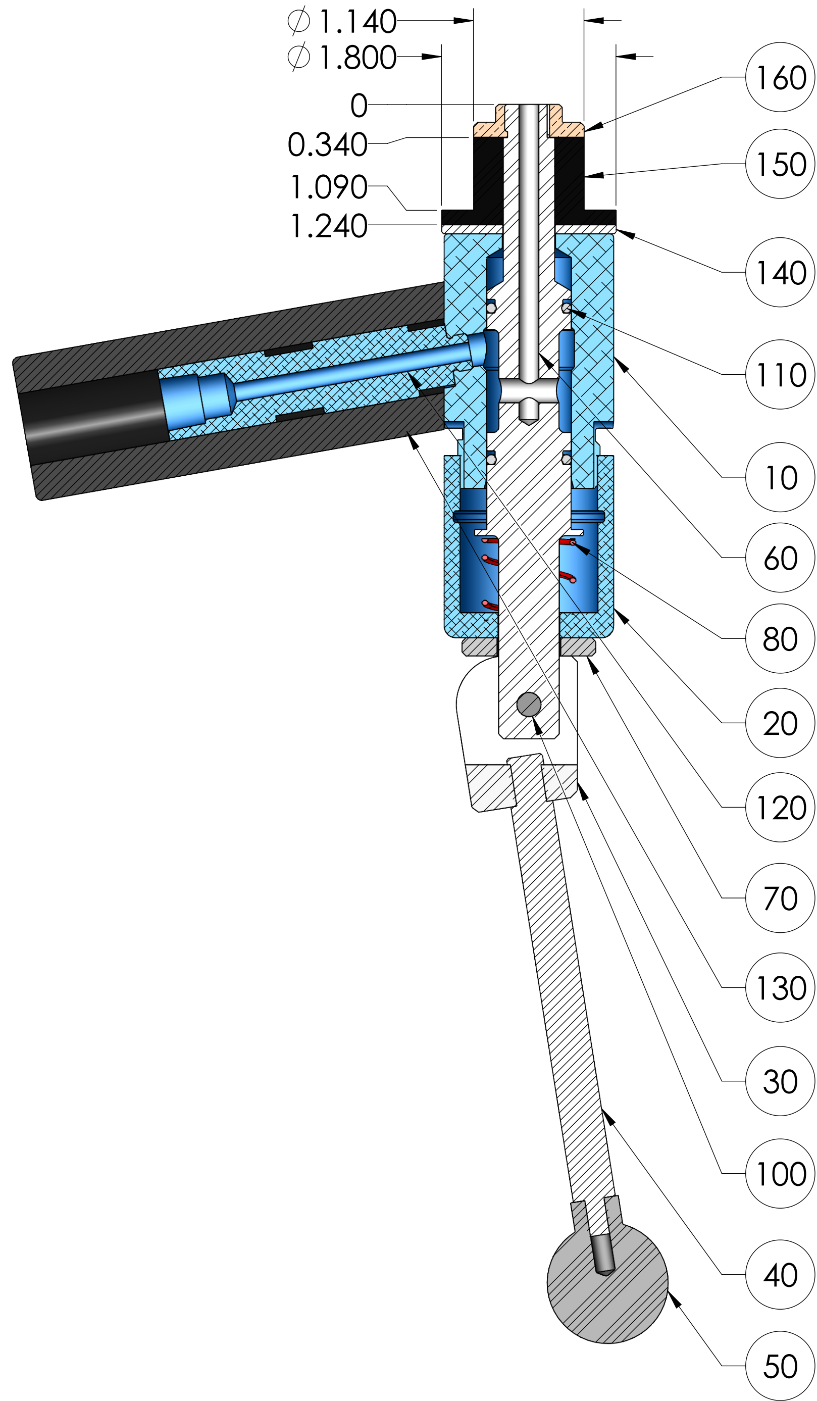
SECTION A-A
