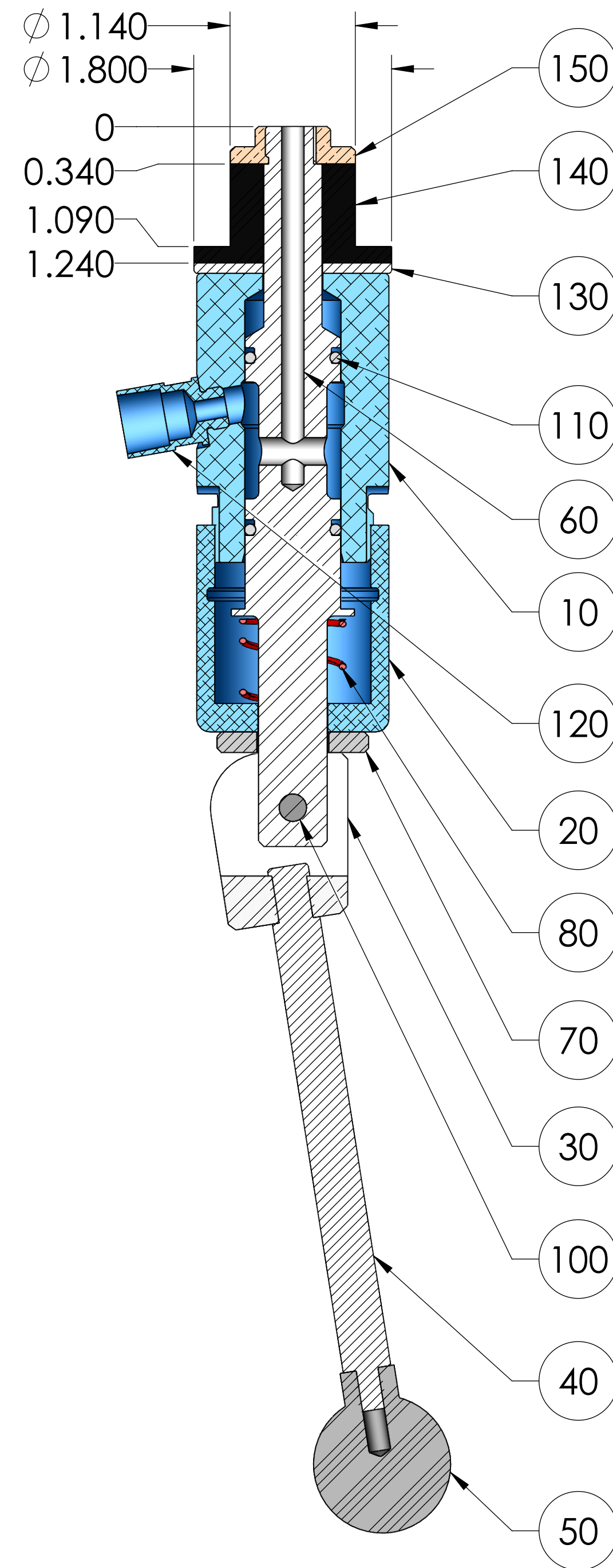
SECTION A-A
