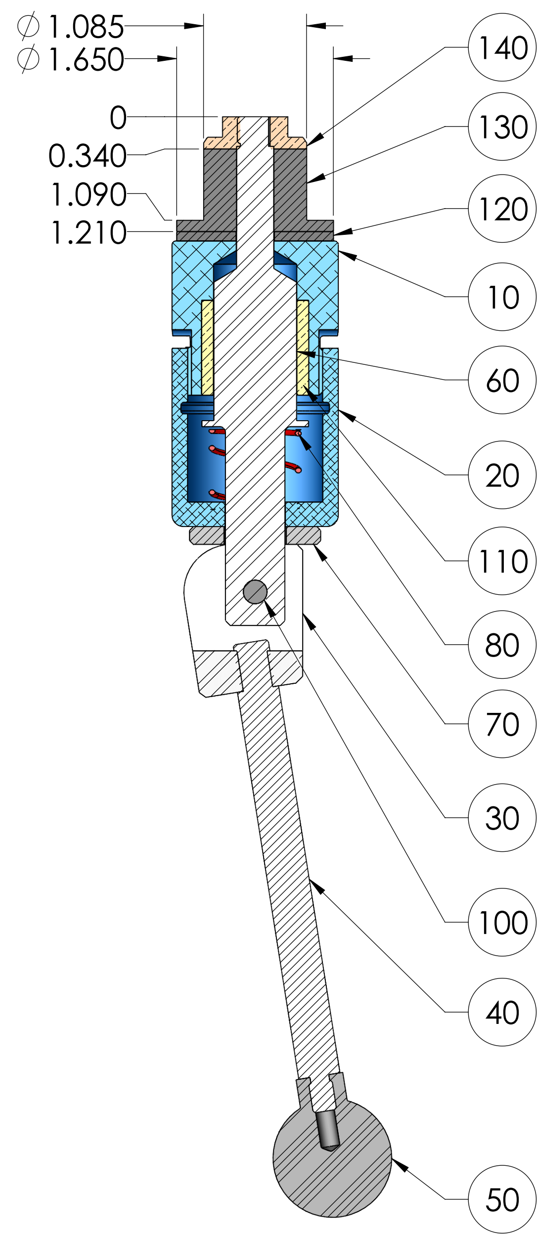
SECTION A-A
