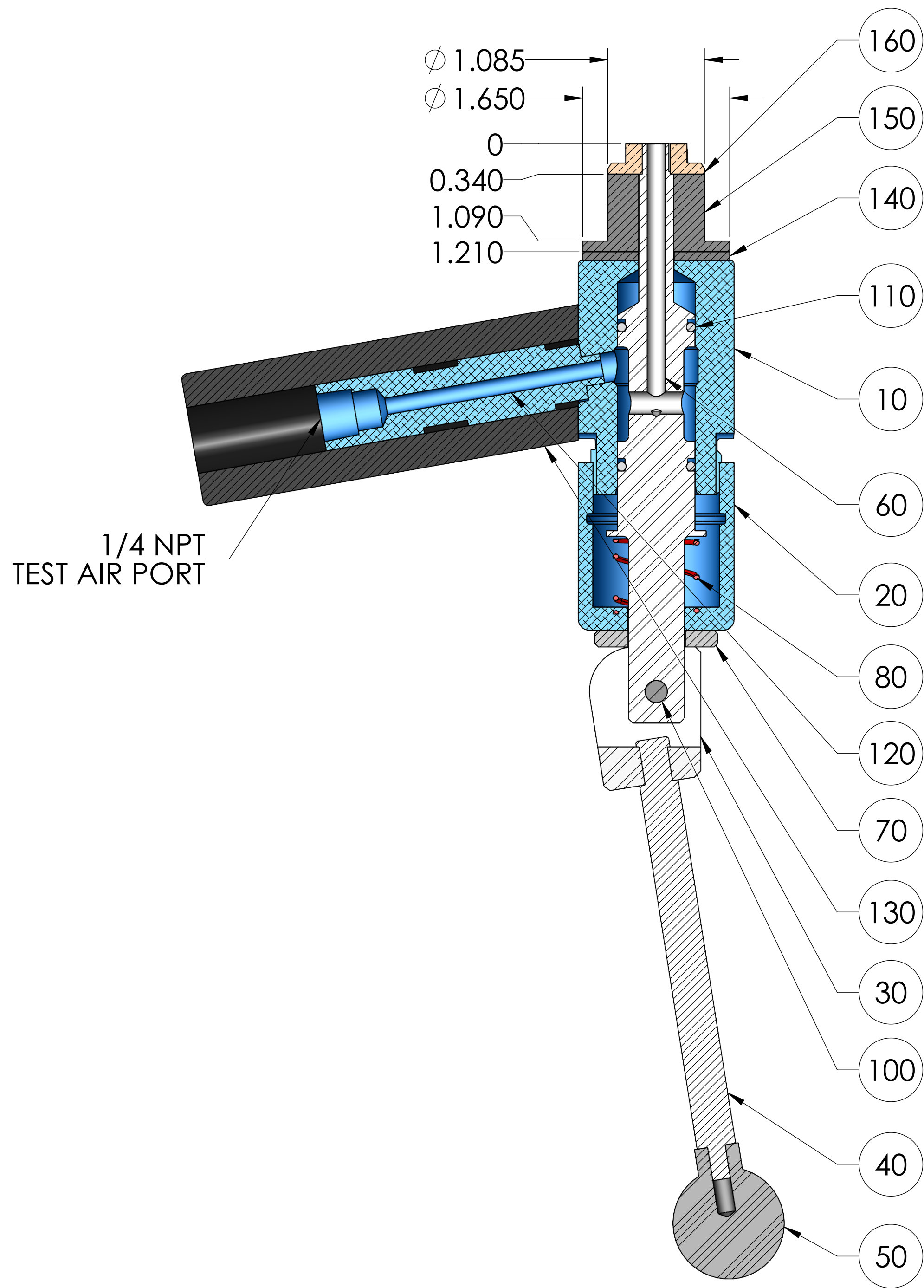
SECTION A-A
