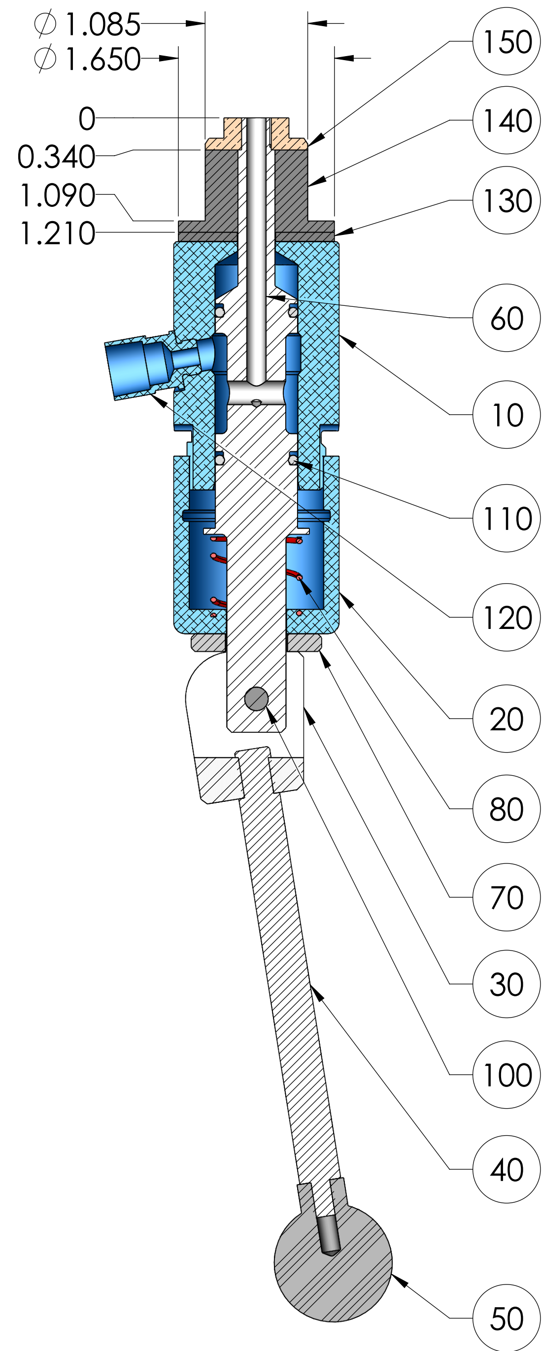
SECTION A-A
