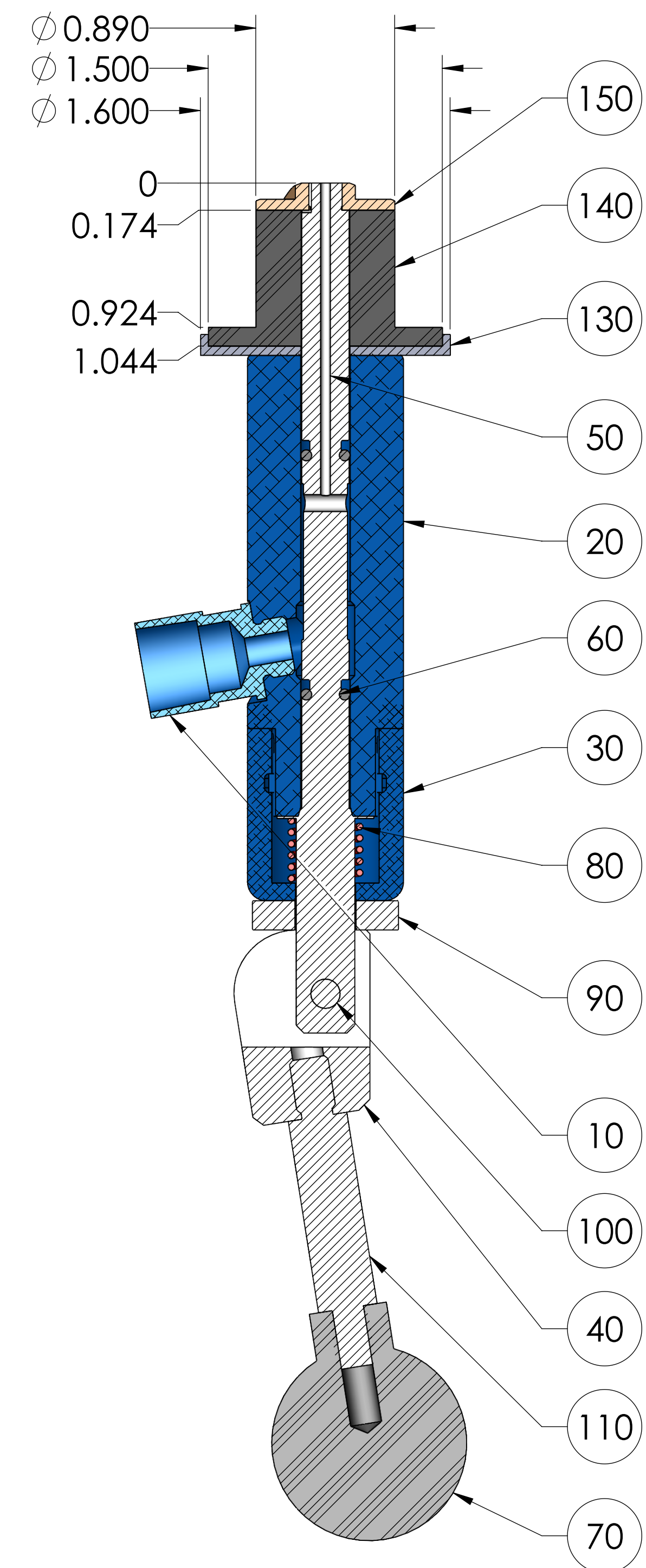
SECTION A-A SCALE 1.5 : 1
