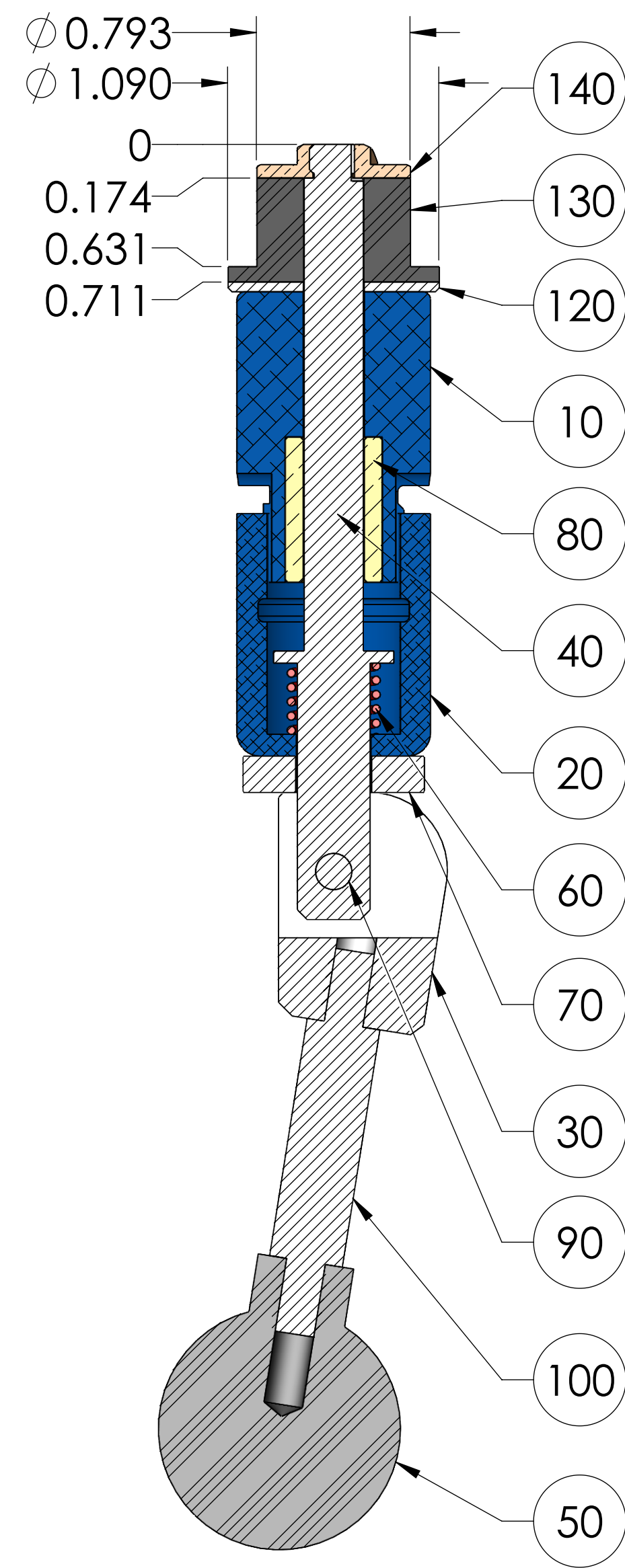
SECTION A-A SCALE 1.5 : 1
