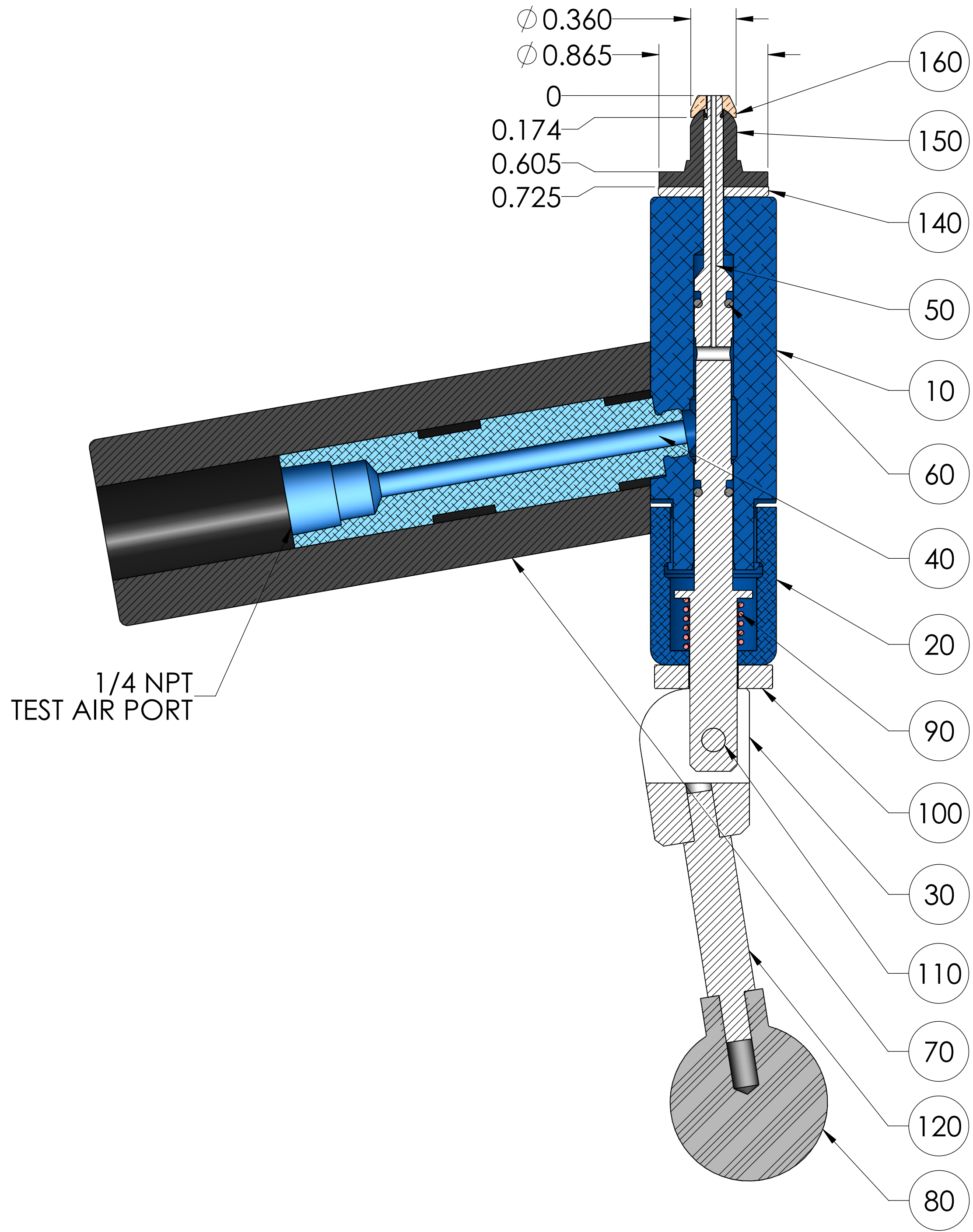
SECTION A-A SCALE 1.5 : 1
