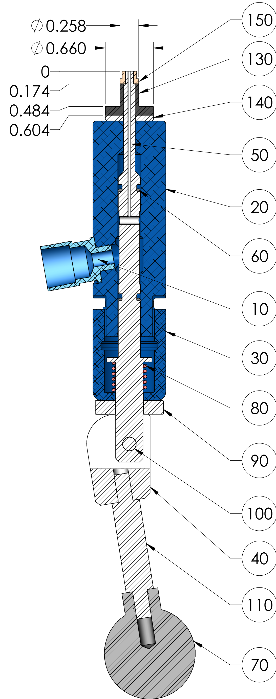
SECTION A-A SCALE 3 : 2
