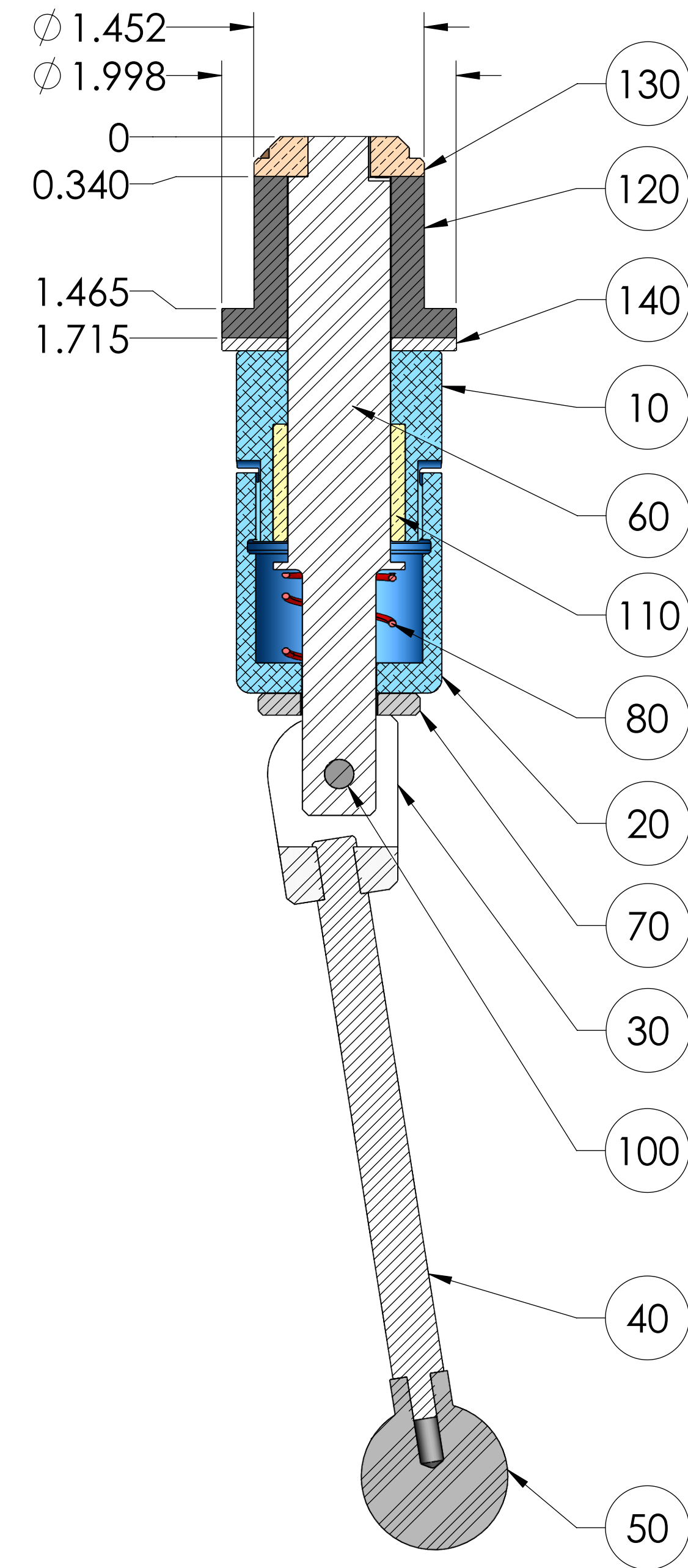
SECTION A-A
