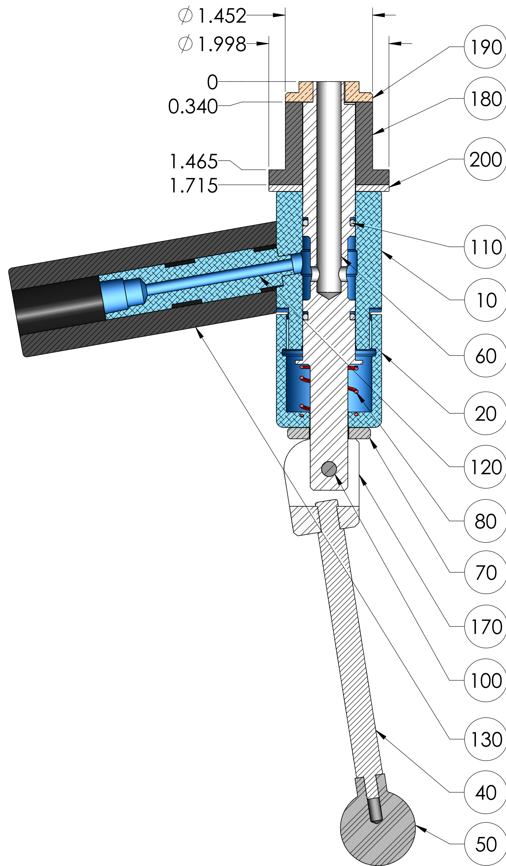
SECTION A-A
