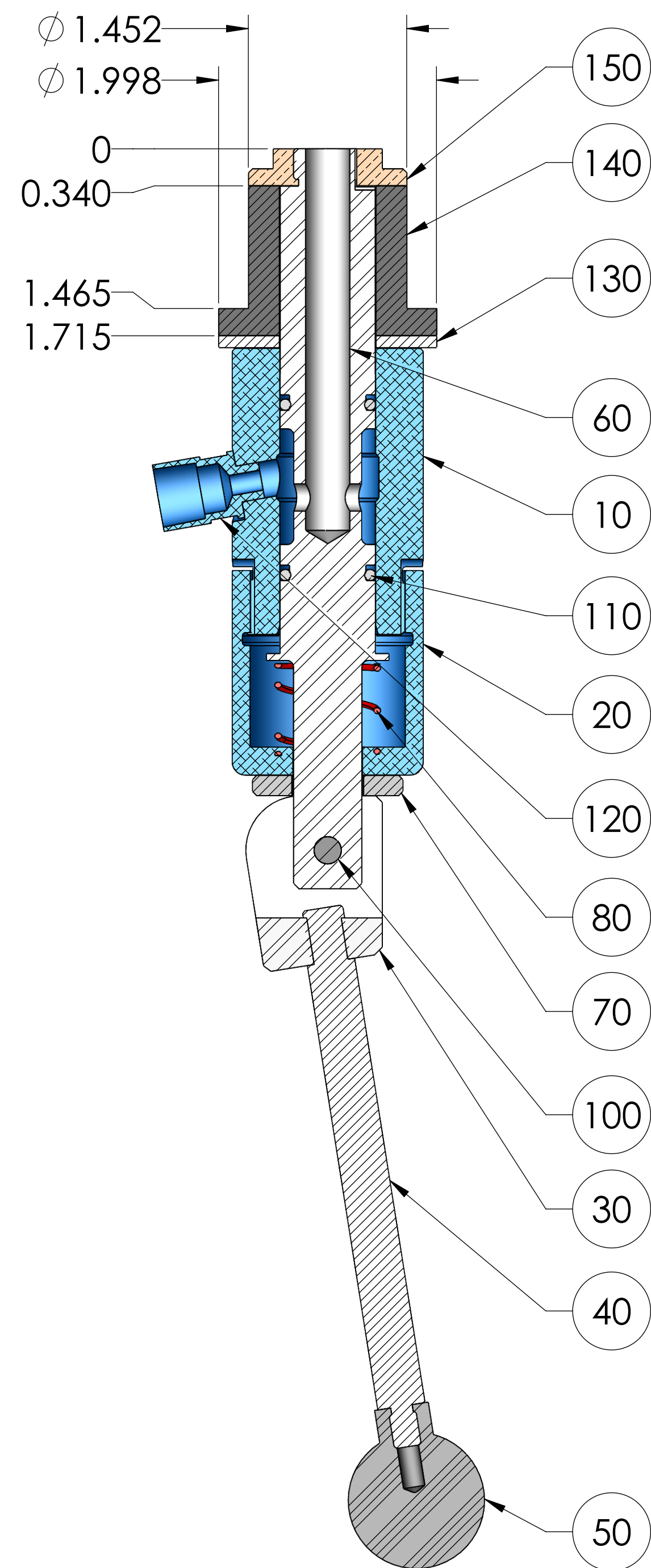
SECTION A-A
