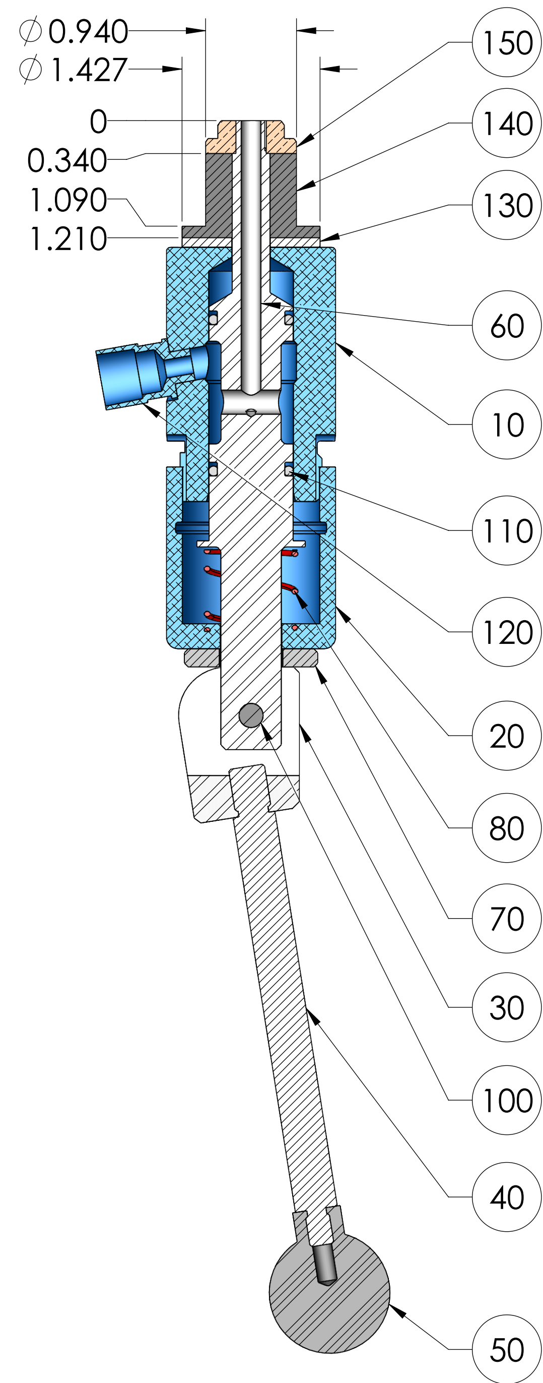
SECTION A-A
