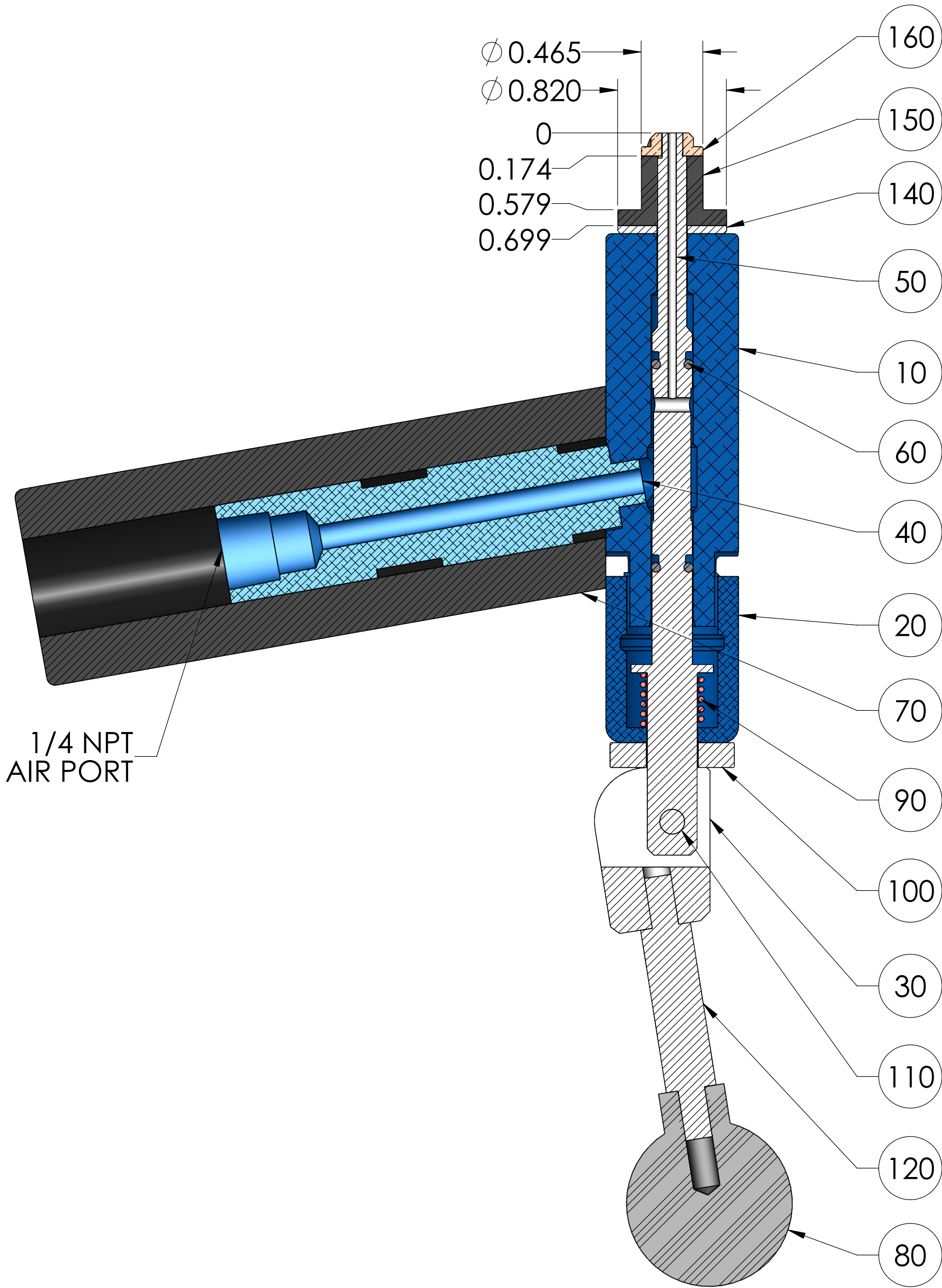
SECTION A-A SCALE 1.5 : 1
