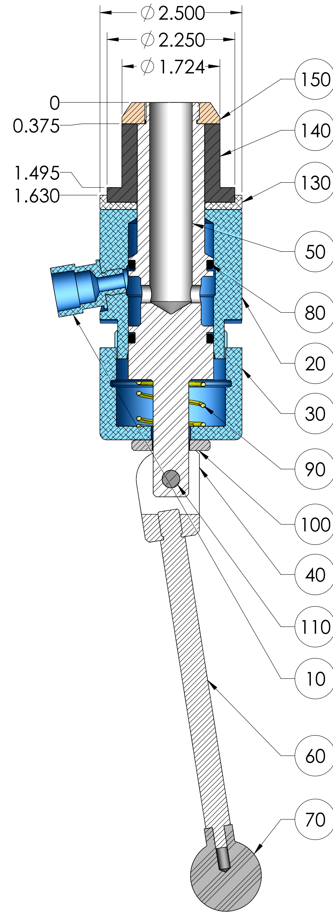
SECTION A-A SCALE 1 : 1
